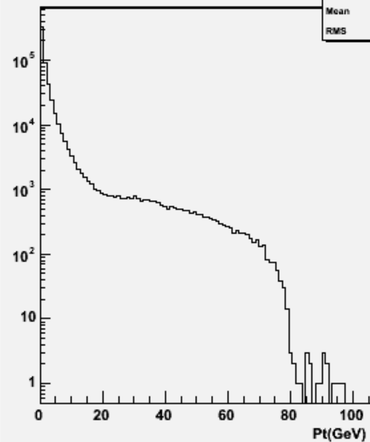
Particle Pt : w104472 e1e1h_o
