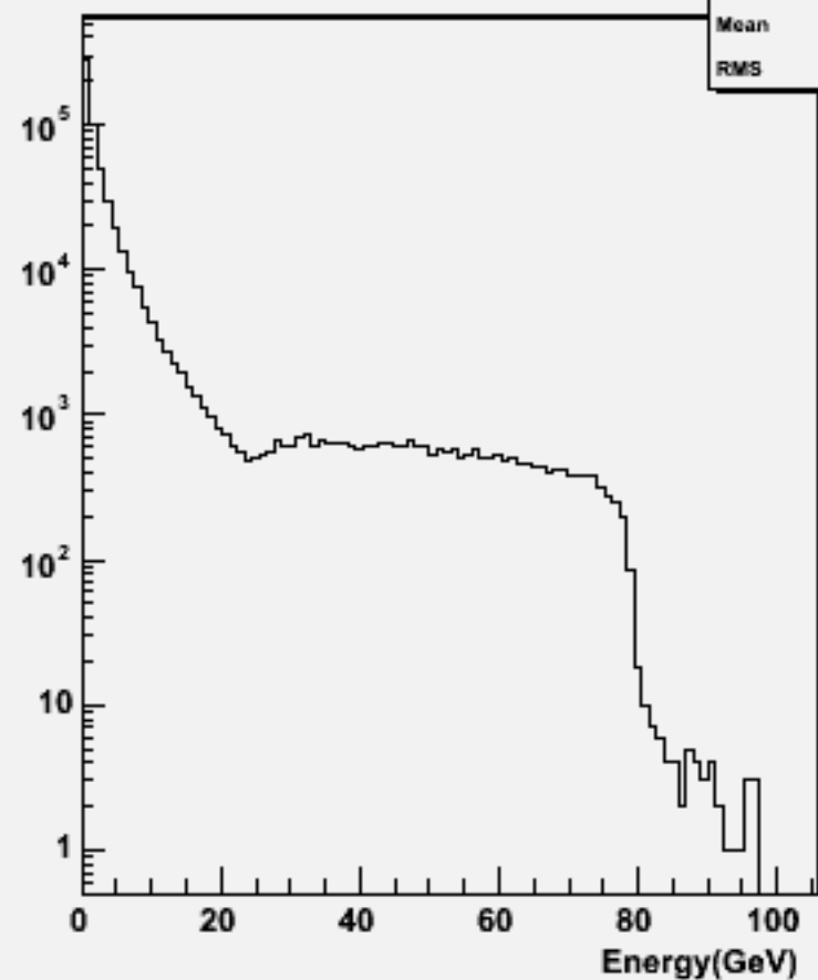
Particle Energy : w104472 e1e1h_o
