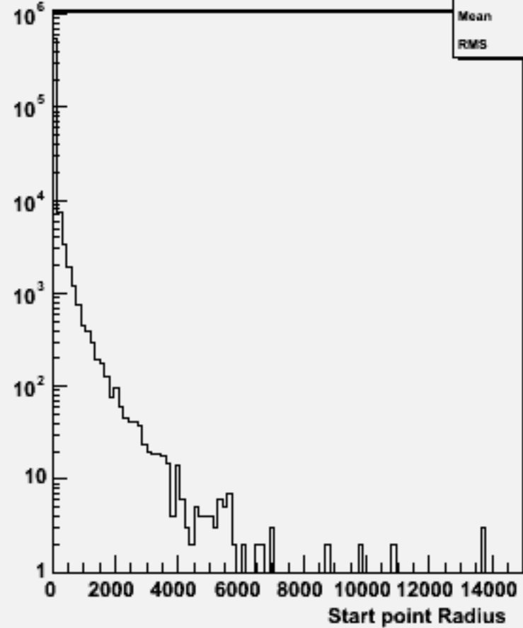
Start point R : w104472 e1e1h_o
