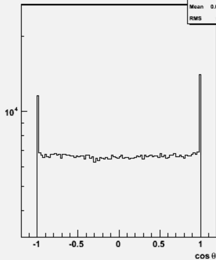
Particle cos \theta : w104472 e1e1h_o
