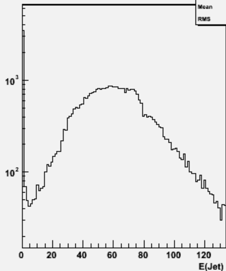
Jet energies(All jets)w104472 e1e1h_o
