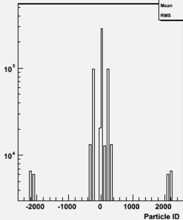
Particle ID : w104472 e1e1h_o
