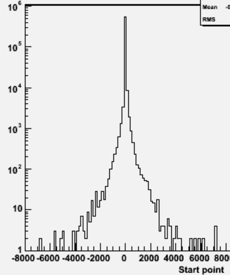
Start point Z : w104472 e1e1h_o
