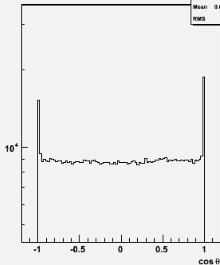
Particle cos \theta : w104471 e1e1h_o
