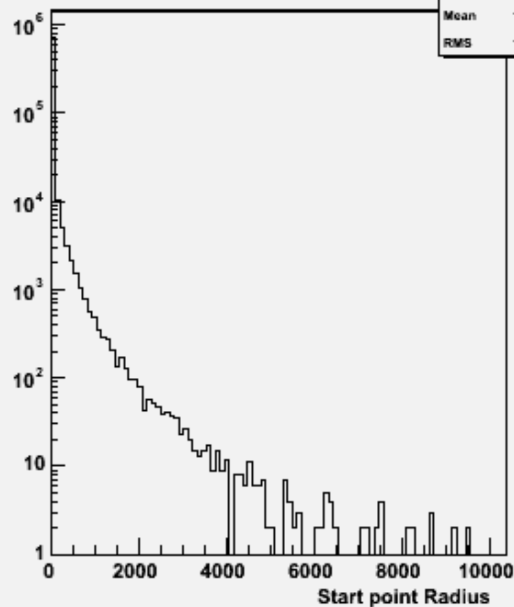
Start point R : w104471 e1e1h_o
