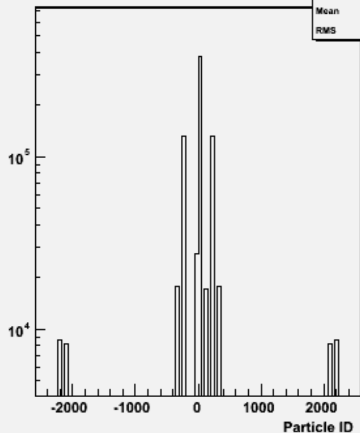
Particle ID : w104471 e1e1h_o
