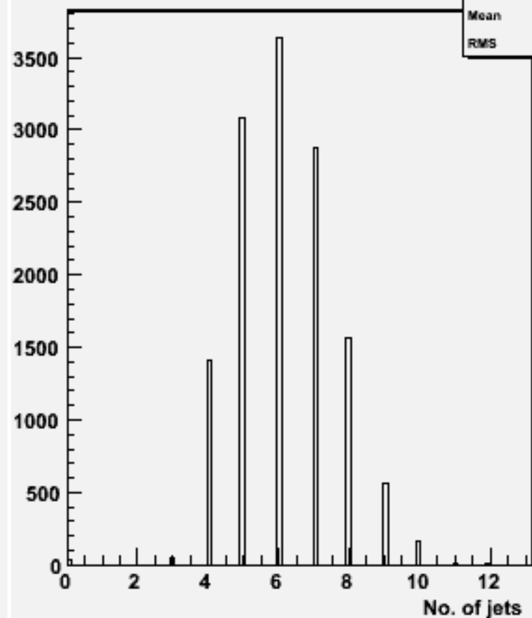
No. jets (ycut=0.001) : w104471 e1e1h_o
