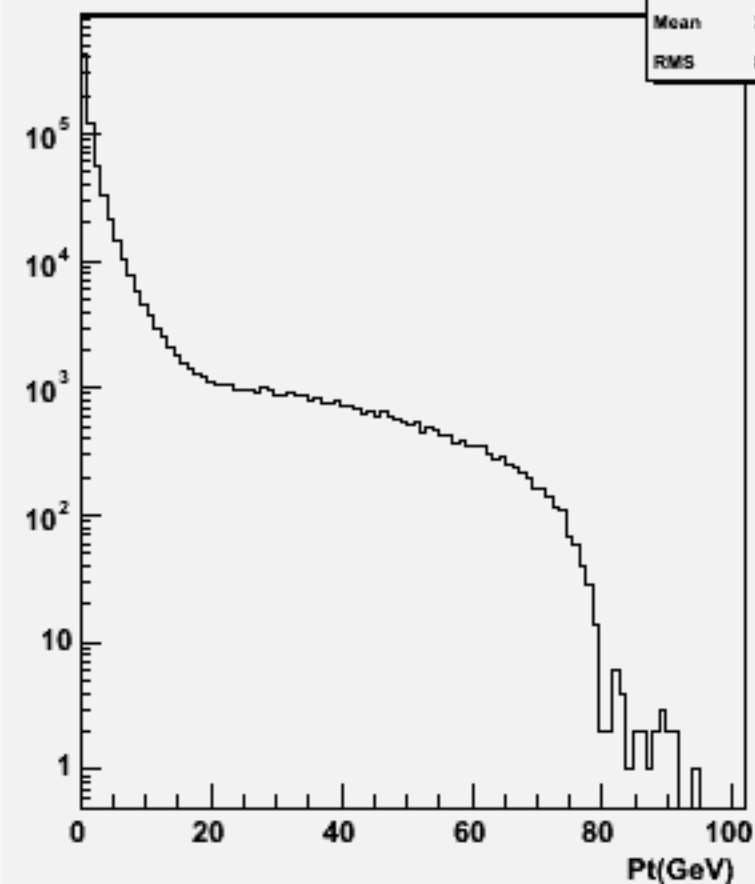
Particle Pt : w104471 e1e1h_o
