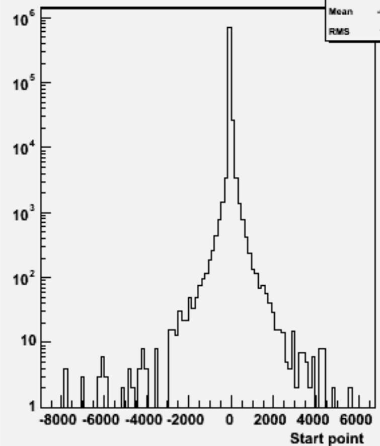
Start point Z : w104471 e1e1h_o
