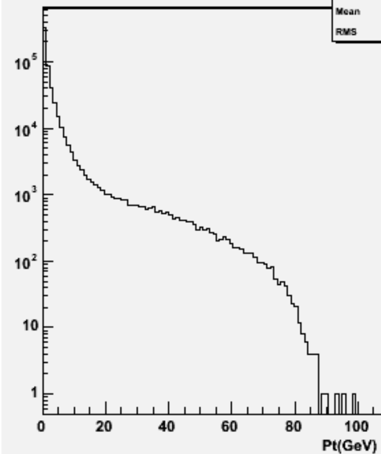
Particle Pt : w104470 e1e1h_o
