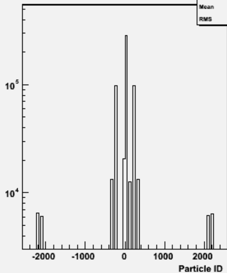
Particle ID : w104470 e1e1h_o
