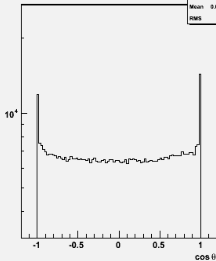
Particle cosθ : w104470 e1e1h_o
