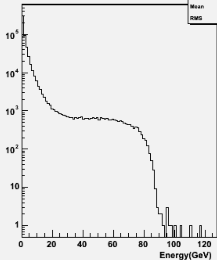
Particle Energy : w104470 e1e1h_o
