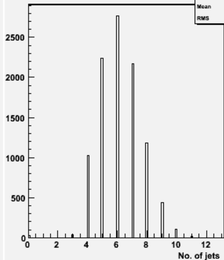
No. jets (ycut=0.001) : w104470 e1e1h_o
