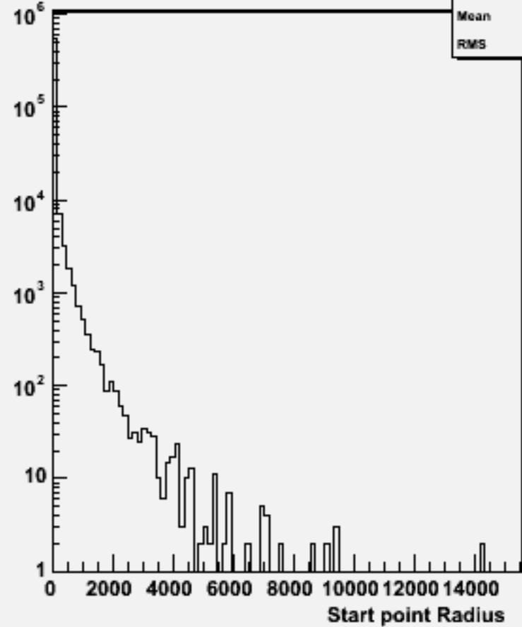
Start point R : w104470 e1e1h_o
