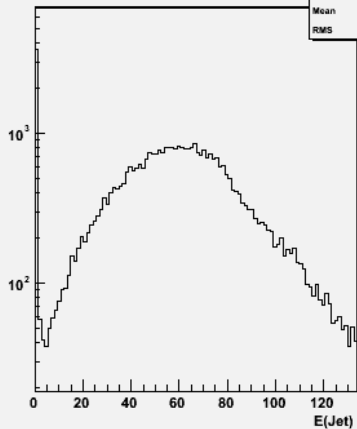
Jet energies(All jets)w104470 e1e1h_o
