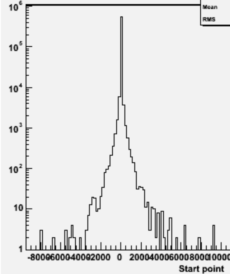
Start point Z : w104470 e1e1h_o
