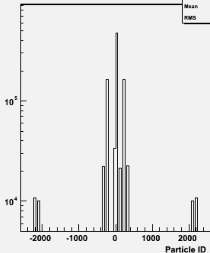
Particle ID : w104460 n3n3h_o
