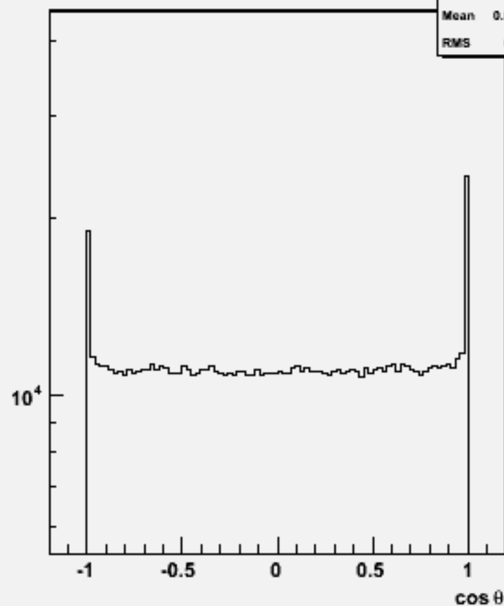
Particle cosθ : w104460 n3n3h_o
