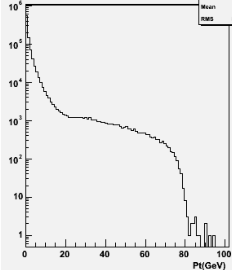
Particle Pt : w104460 n3n3h_o
