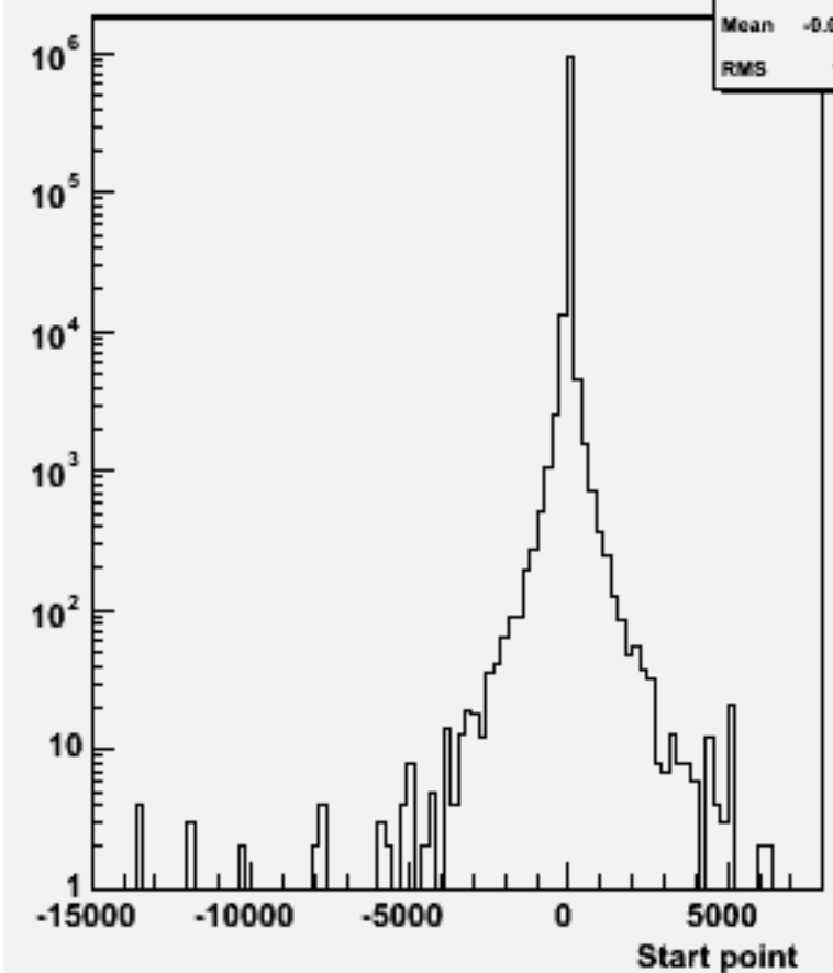
Start point Z : w104460 n3n3h_o
