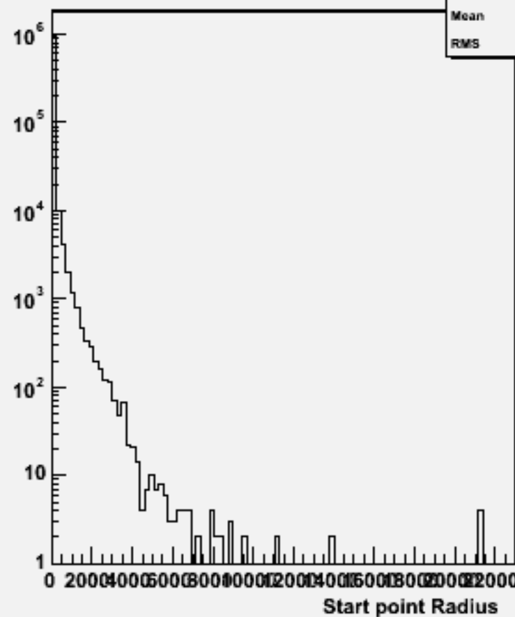
Start point R : w104460 n3n3h_o
