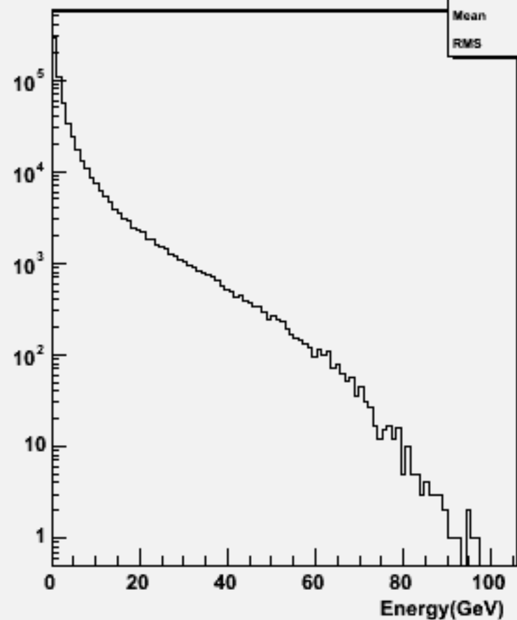
Particle Energy : w104430 e3e3h_o
