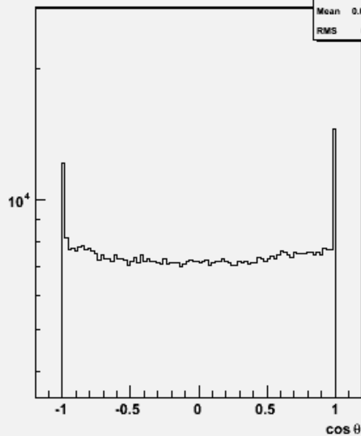
Particle \cos\theta : w104430 e3e3h_o
