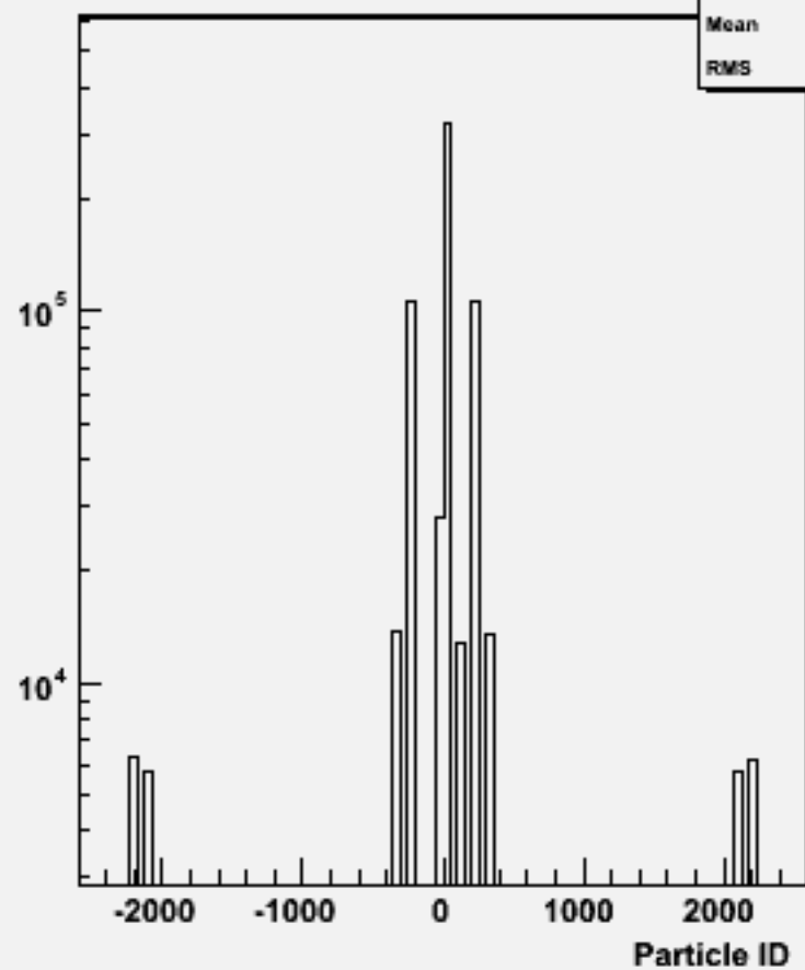
Particle ID : w104430 e3e3h_o
