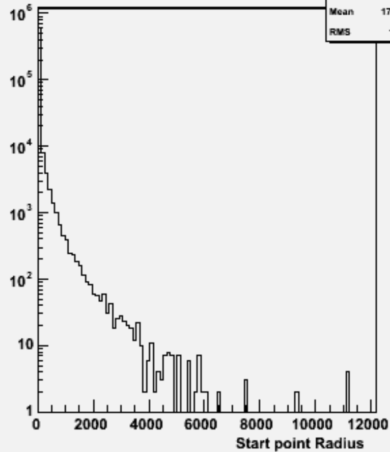
Start point R : w104430 e3e3h_o
