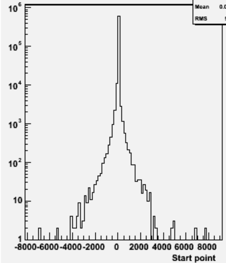
Start point Z : w104430 e3e3h_o
