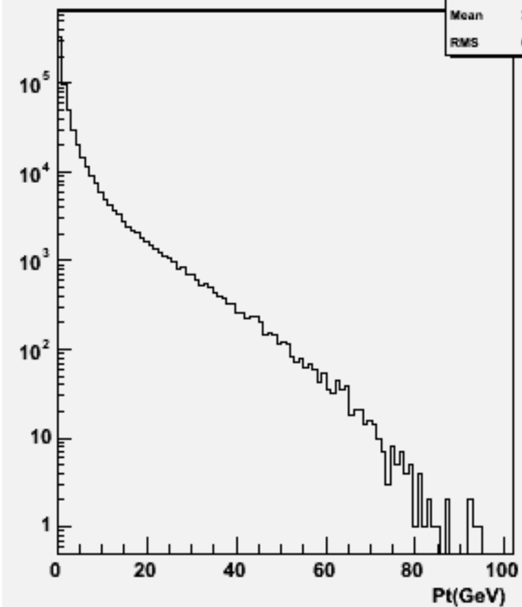
Particle Pt : w104430 e3e3h_o
