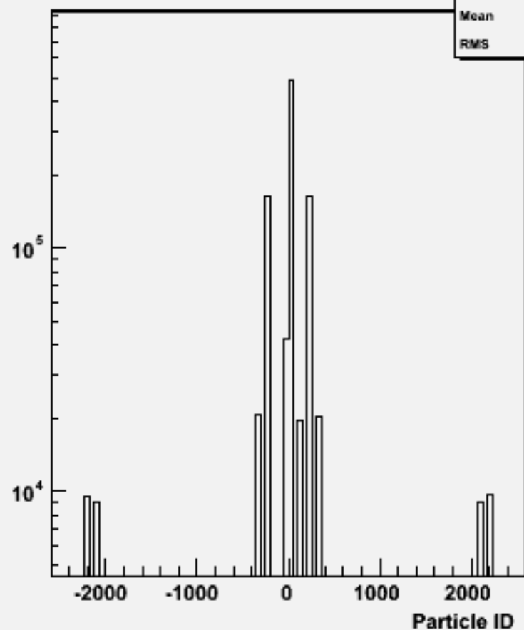
Particle ID : w104429 e3e3h_o
