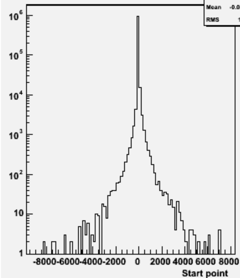
Start point Z : w104429 e3e3h_o
