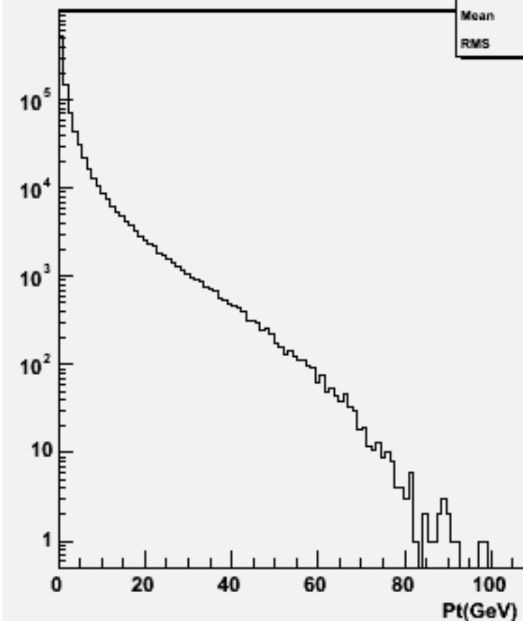
Particle Pt : w104429 e3e3h_o
