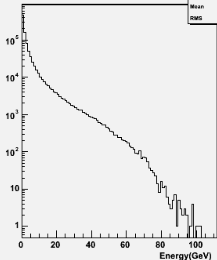
Particle Energy : w104429 e3e3h_o
