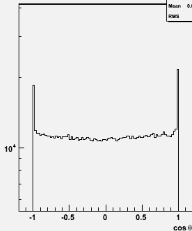
Particle cosθ : w104429 e3e3h_o
