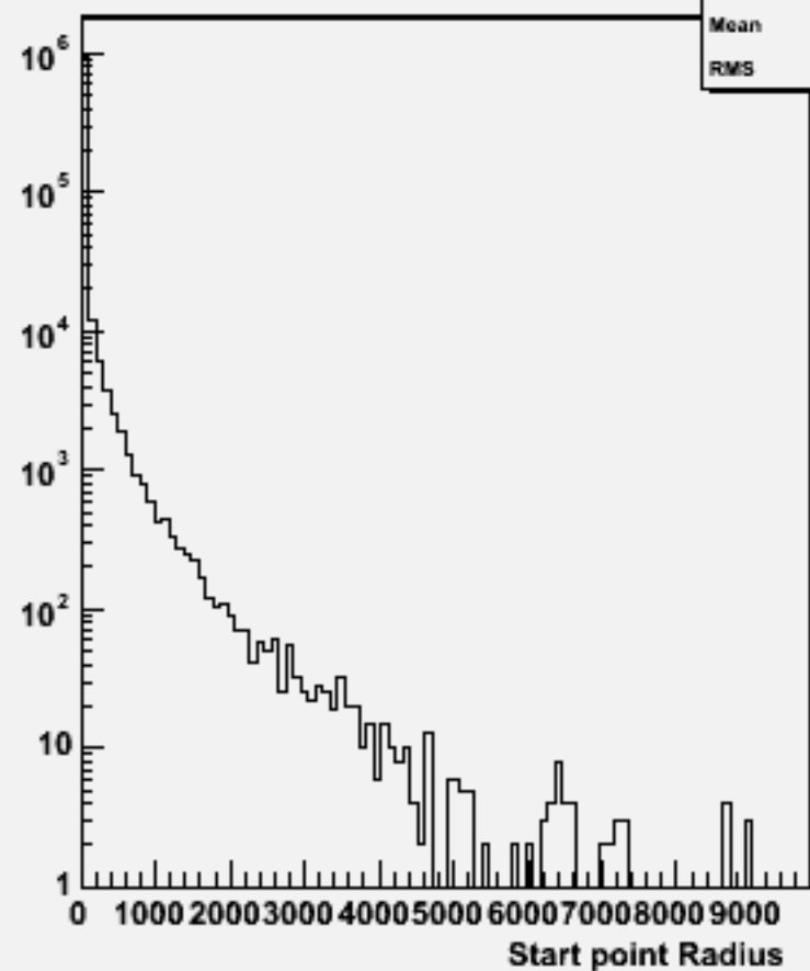
Start point R : w104429 e3e3h_o
