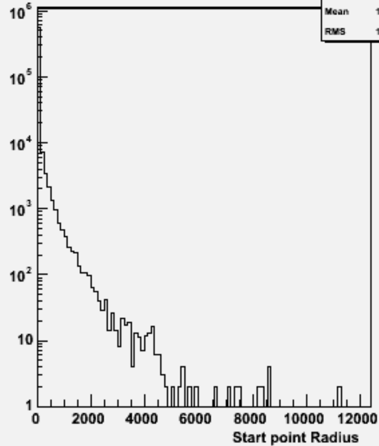
Start point R : w104426 e2e2h_o
