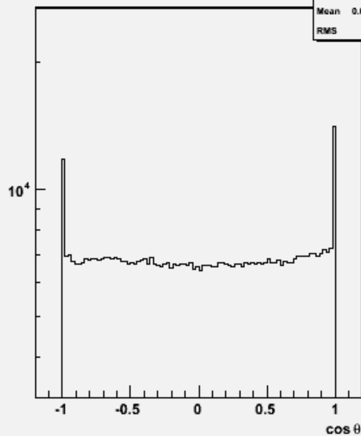
Particle cosθ : w104426 e2e2h_o
