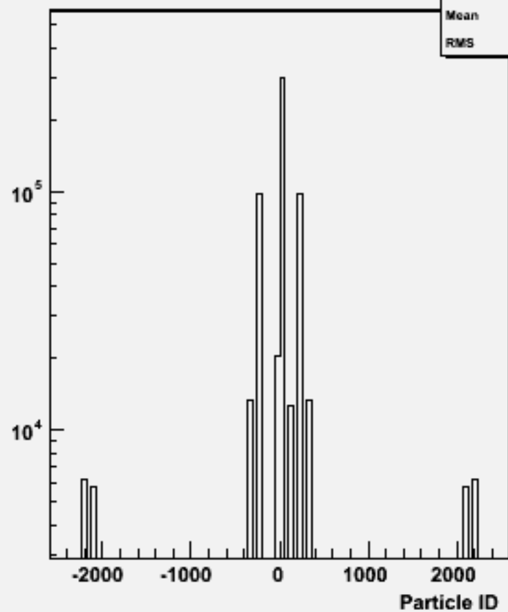
Particle ID : w104426 e2e2h_o
