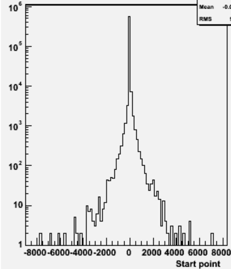
Start point Z : w104426 e2e2h_o
