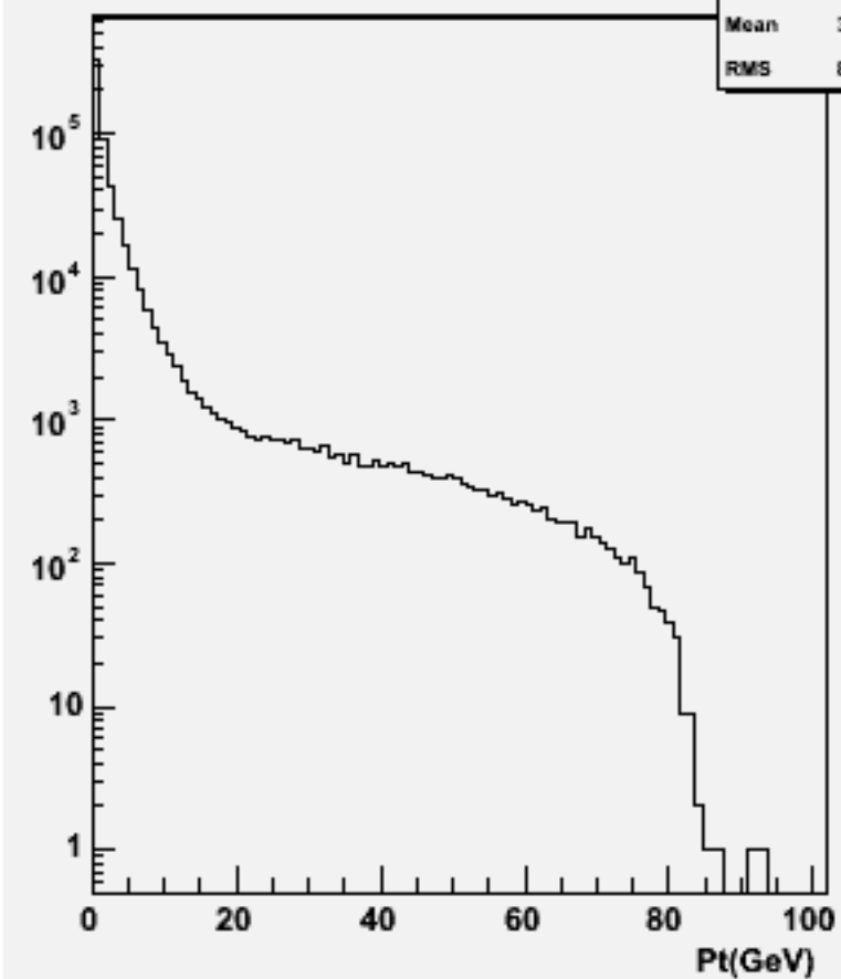
Particle Pt : w104426 e2e2h_o
