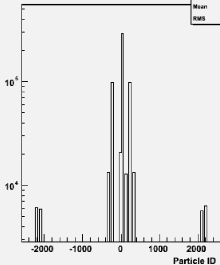
Particle ID : w104423 e1e1h_o
