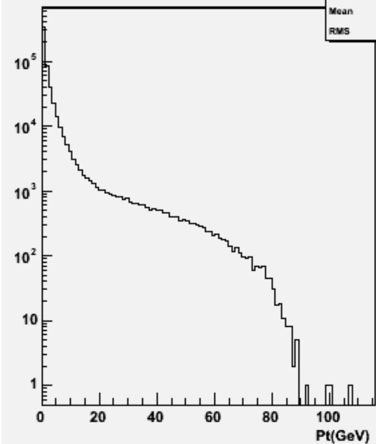
Particle Pt : w104423 e1e1h_o
