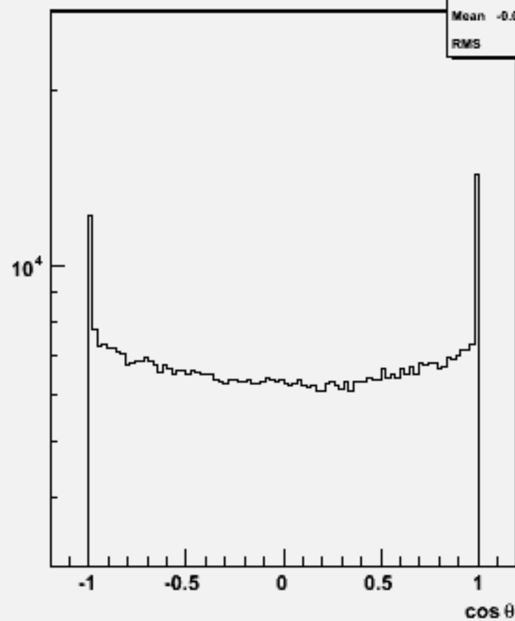
Particle cos \theta : w104423 e1e1h_o
