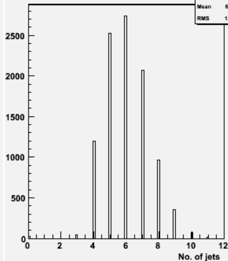
No. jets (ycut=0.001) : w104423 e1e1h_o
