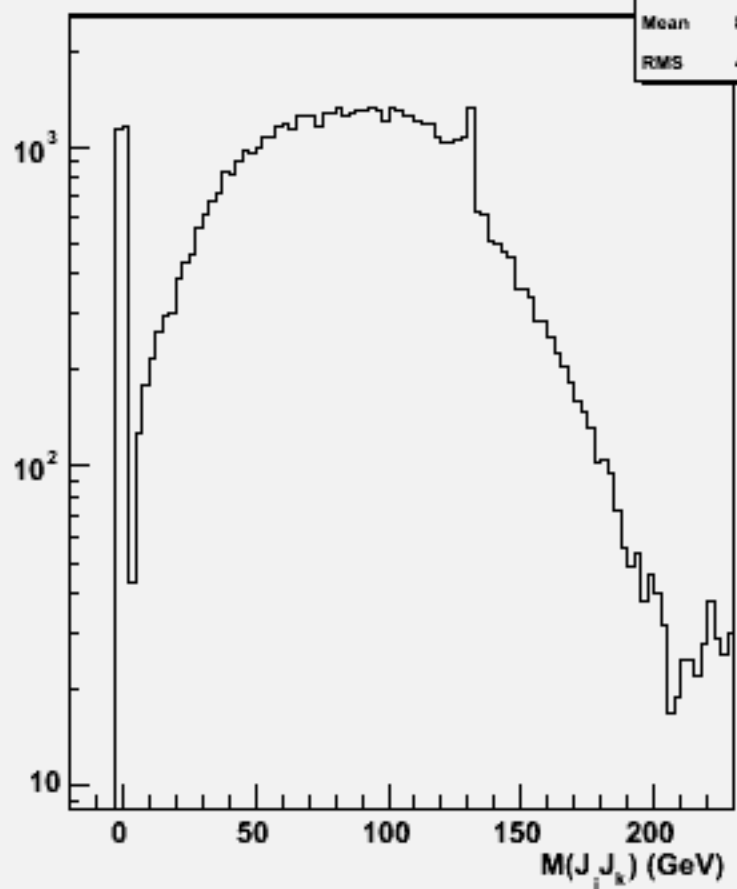
2jets mass(All comb)w104423 e1e1h_o
