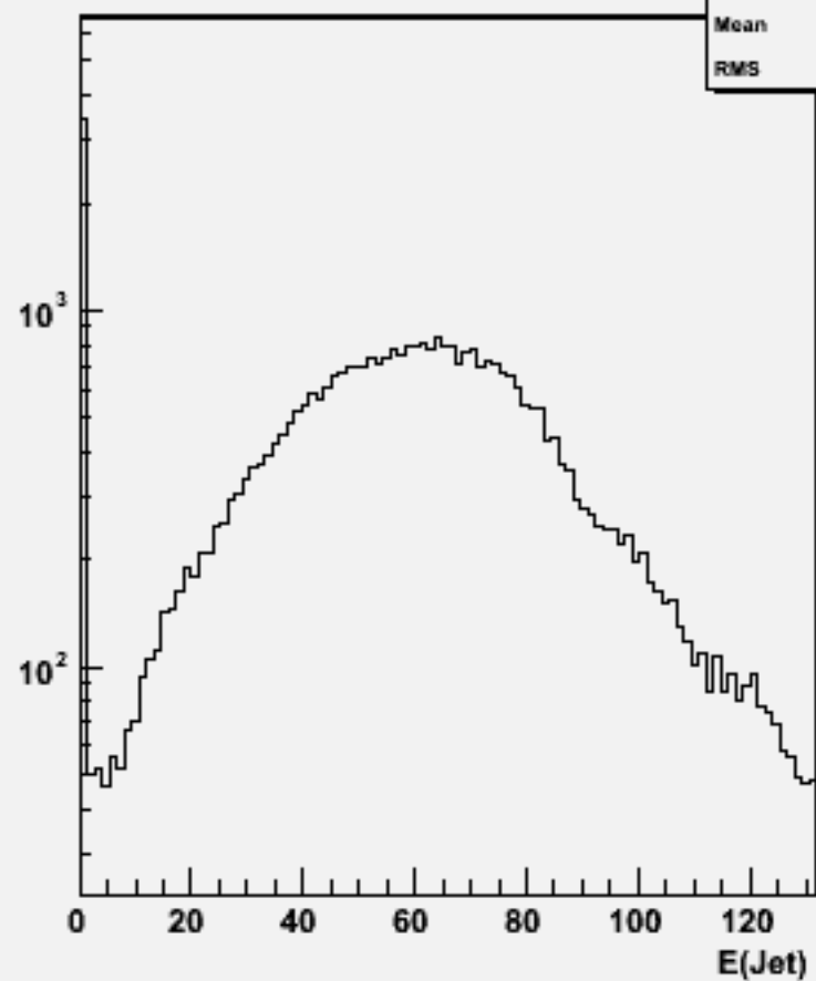
Jet energies(All jets)w104423 e1e1h_o
