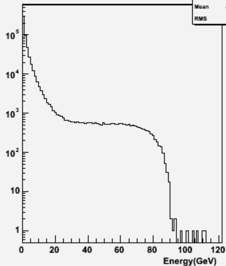
Particle Energy : w104423 e1e1h_o
