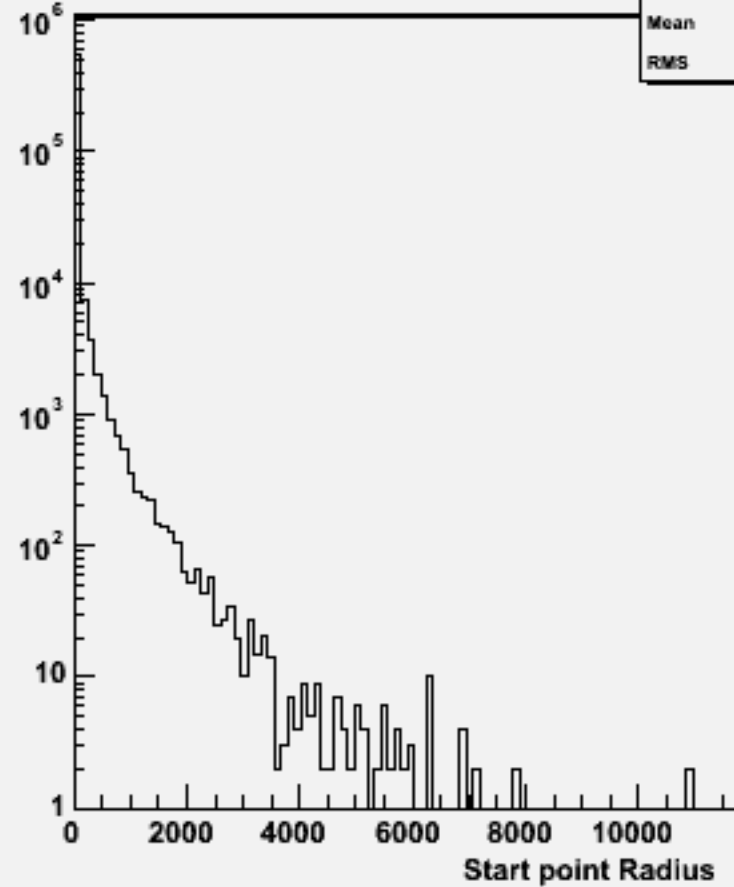
Start point R : w104423 e1e1h_o
