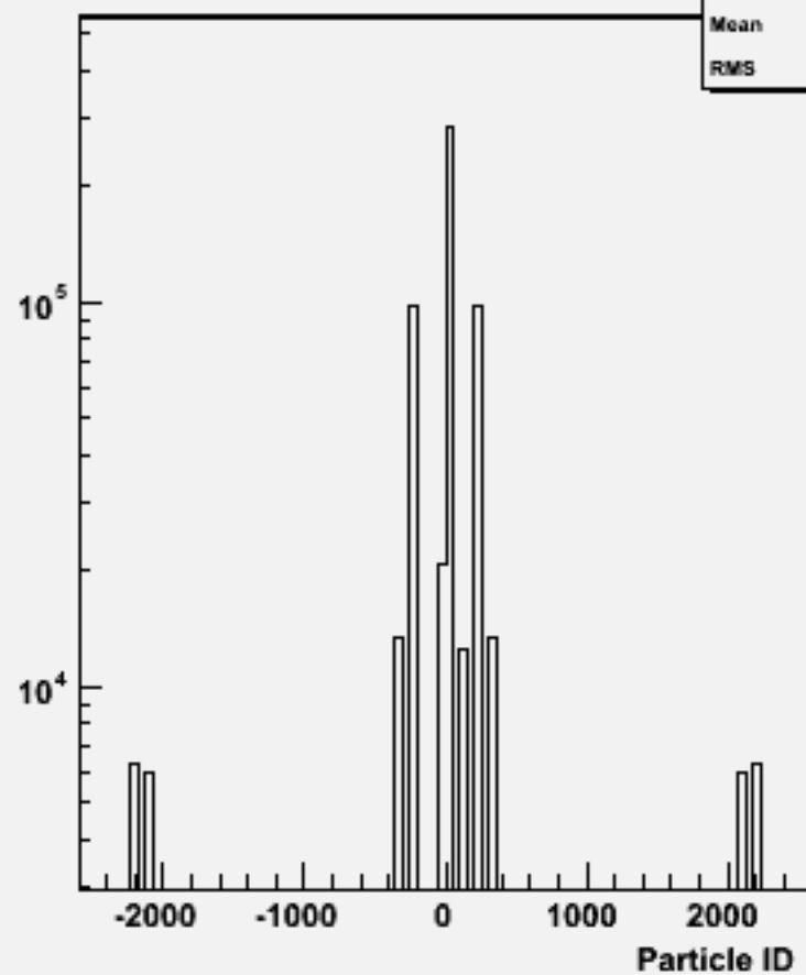
Particle ID : w104422 e1e1h_o
