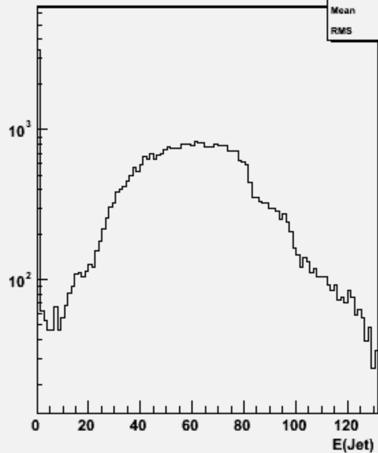
Jet energies(All jets)w104422 e1e1h_o
