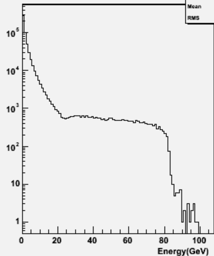
Particle Energy : w104422 e1e1h_o
