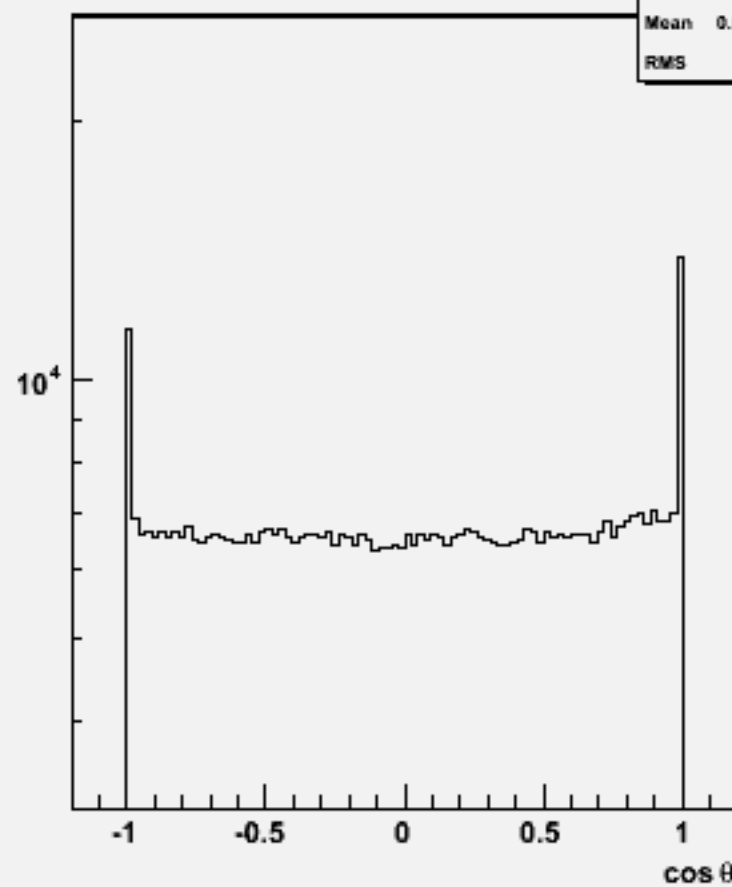
Particle \cos\theta : w104422 e1e1h_o
