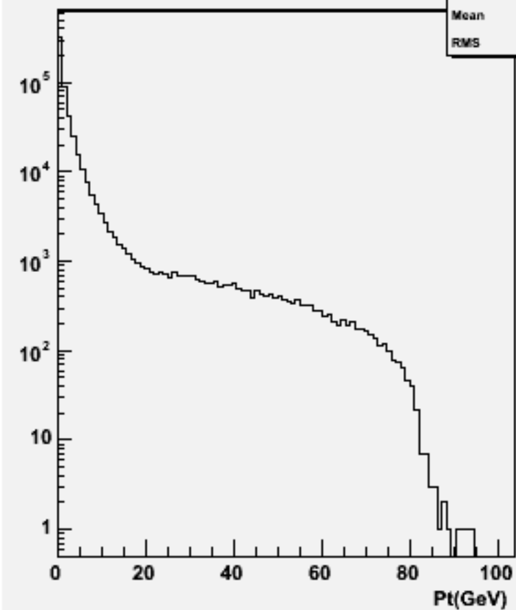
Particle Pt : w104422 e1e1h_o
