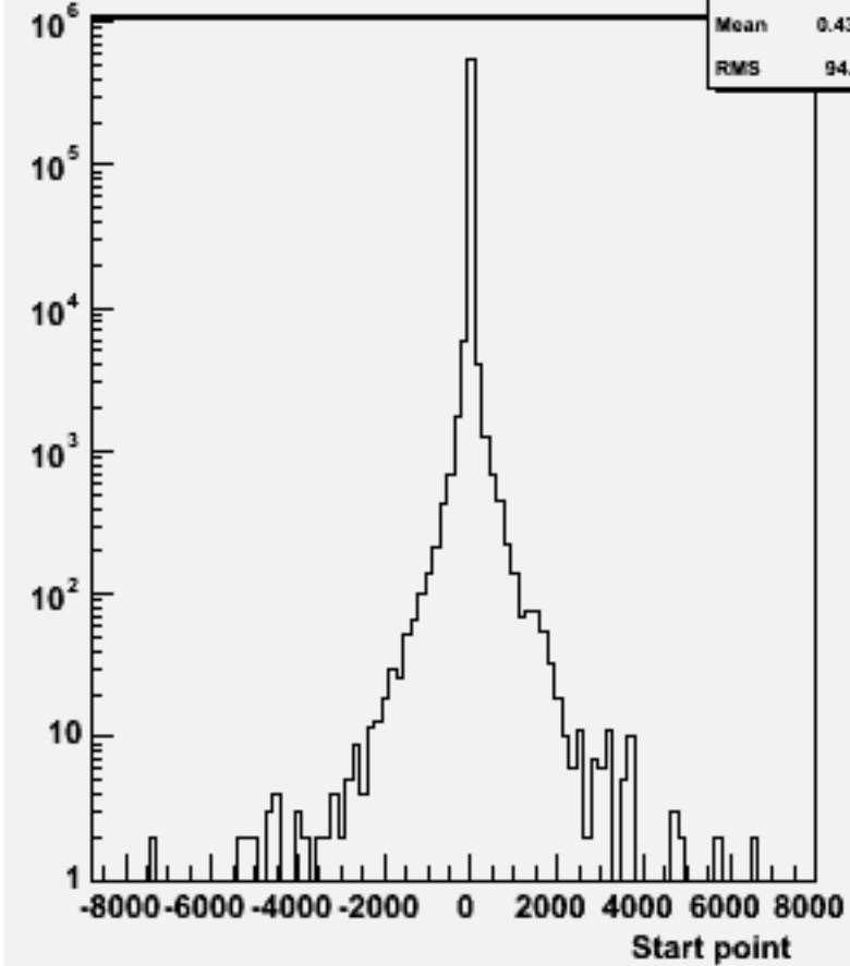
Start point Z : w104422 e1e1h_o
