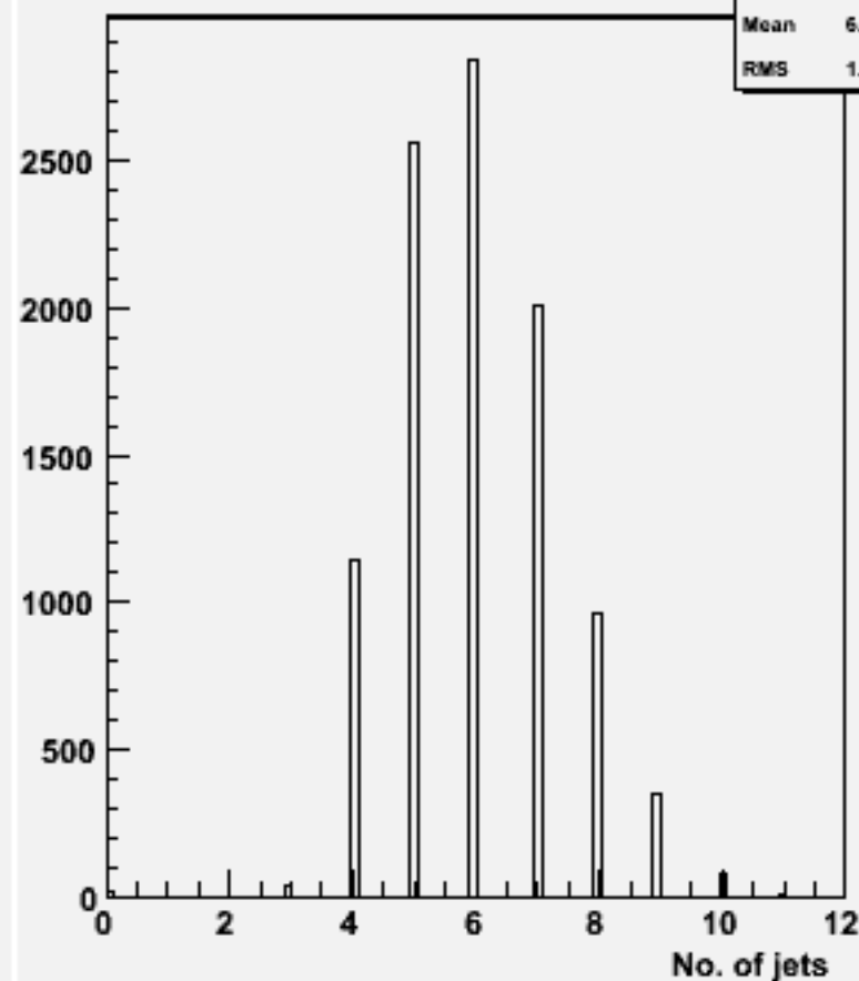
No. jets (ycut=0.001) : w104422 e1e1h_o
