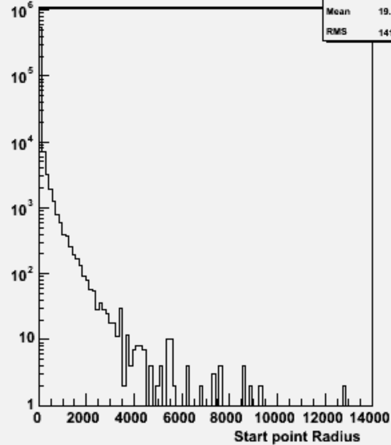
Start point R : w104422 e1e1h_o
