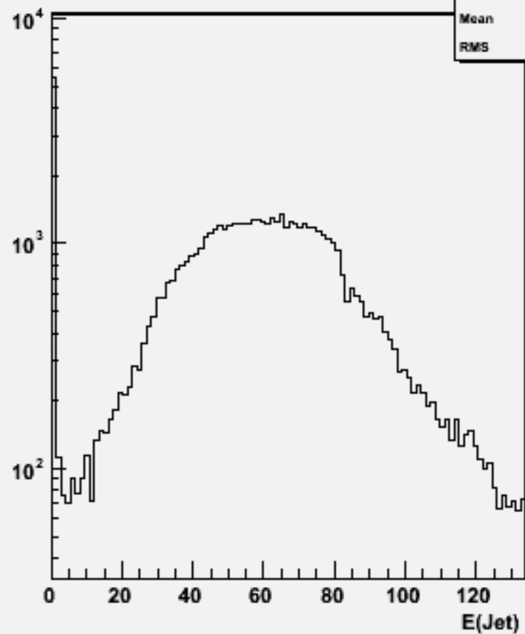
Jet energies(All jets)w104421 e1e1h_o
