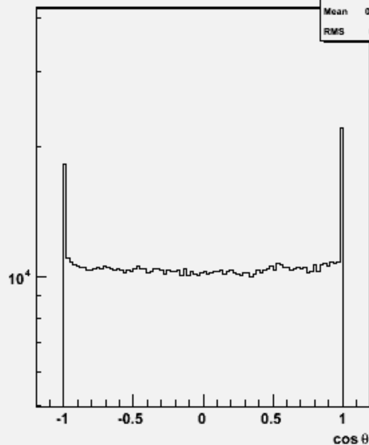
Particle cosθ : w104421 e1e1h_o
