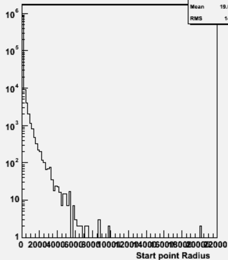
Start point R : w104421 e1e1h_o
