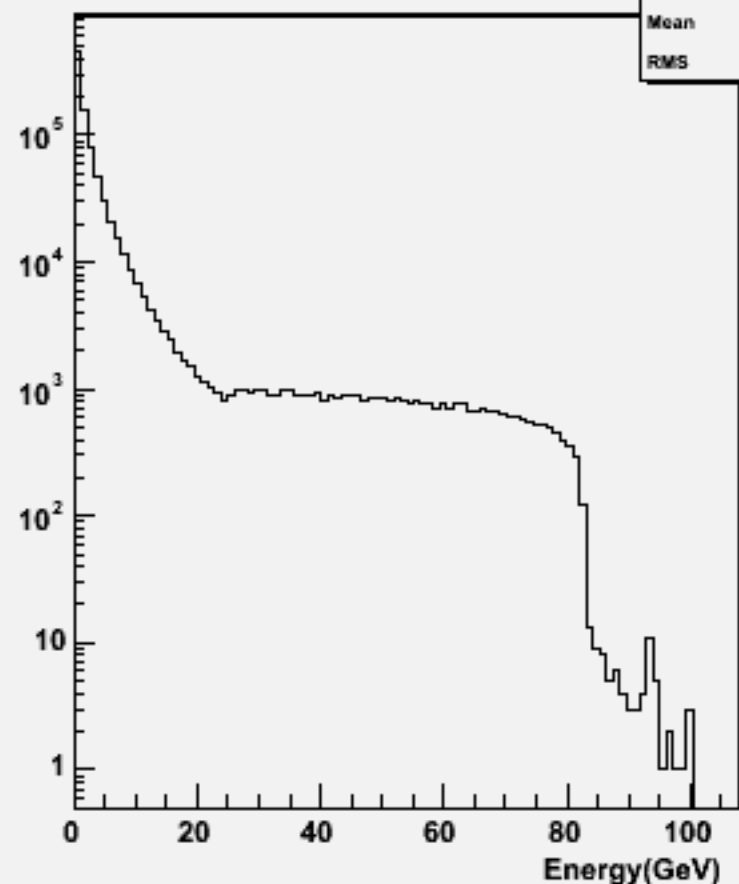
Particle Energy : w104421 e1e1h_o
