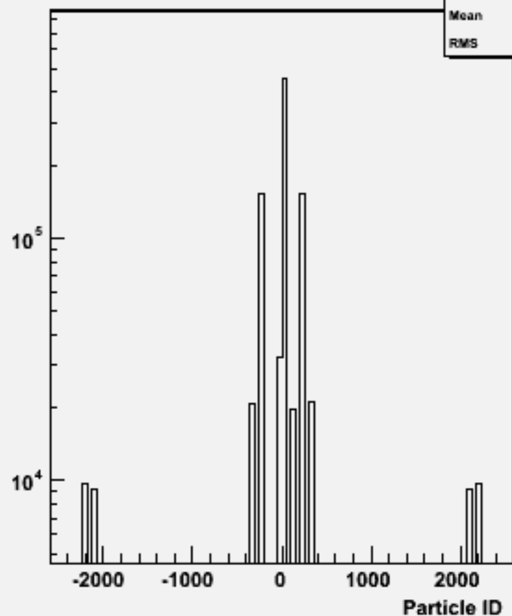
Particle ID : w104421 e1e1h_o
