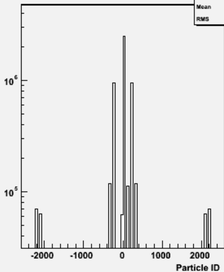
Particle ID : w104413 uuh_o
