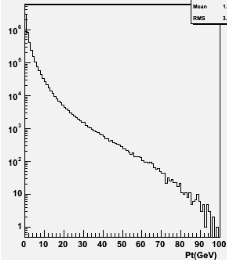
Particle Pt : w104413 uuh_o
