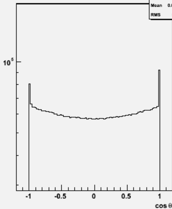
Particle \cos\theta : w104413 uuh_o
