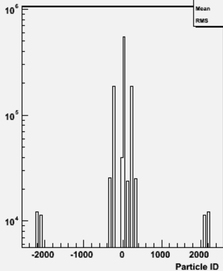
Particle ID : w104410 n3n3h_o
