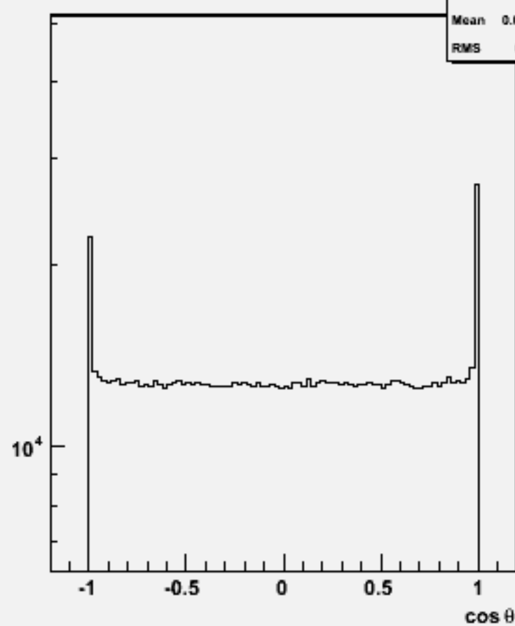
Particle \cos\theta : w104410 n3n3h_o
