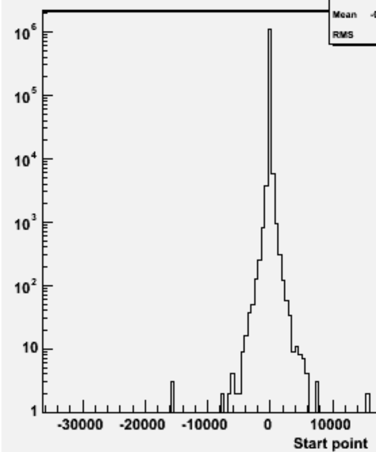
Start point Z : w104410 n3n3h_o
