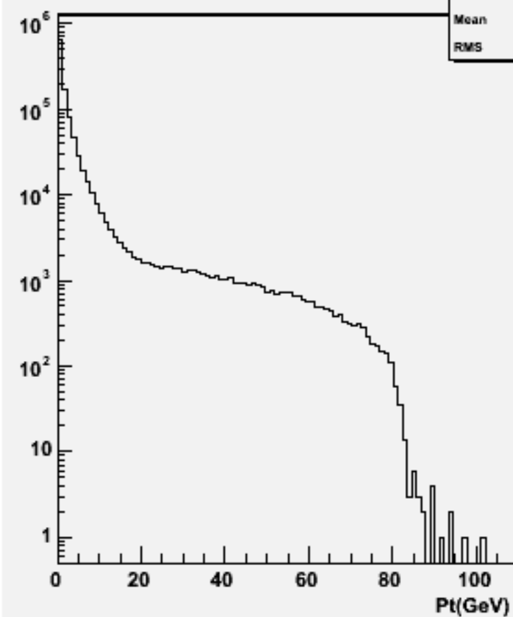
Particle Pt : w104410 n3n3h_o
