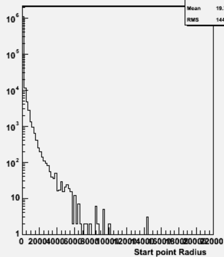
Start point R : w104410 n3n3h_o
