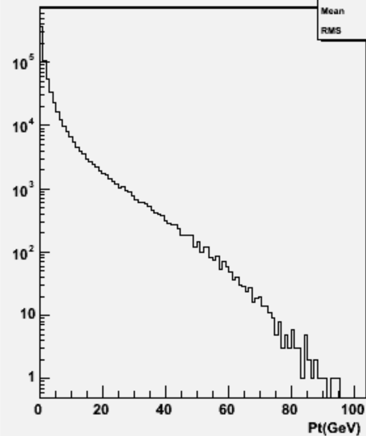
Start point Z : w104380 e3e3h_o
