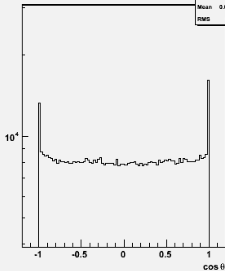
Particle cos \theta : w104380 e3e3h_o
