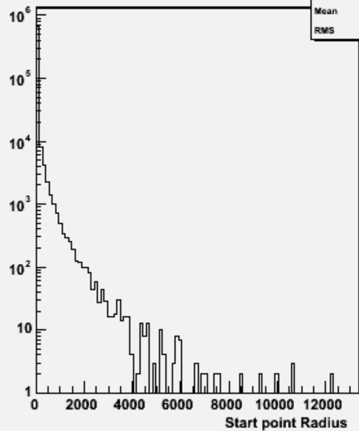
Start point R : w104380 e3e3h_o
