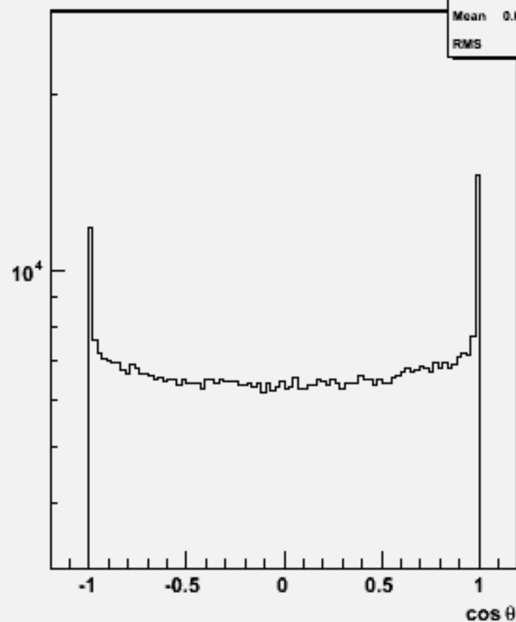
Particle cosθ : w104370 e1e1h_o
