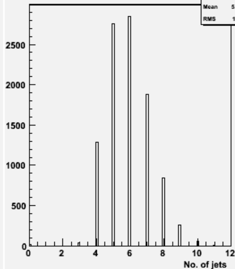
No. jets (ycut=0.001) : w104370 e1e1h_o
