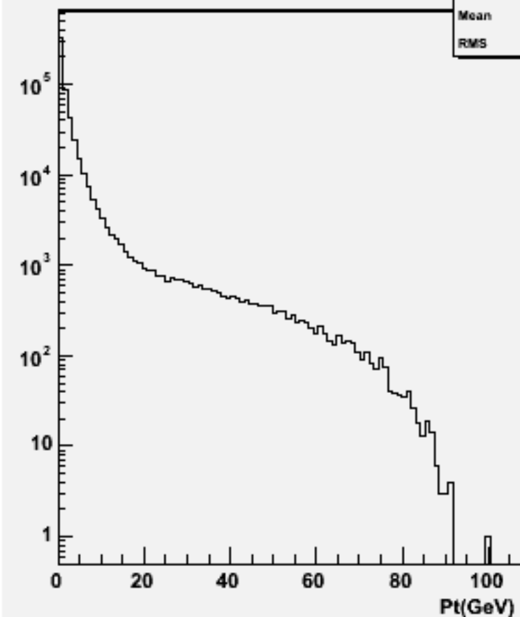
Particle Pt : w104370 e1e1h_o
