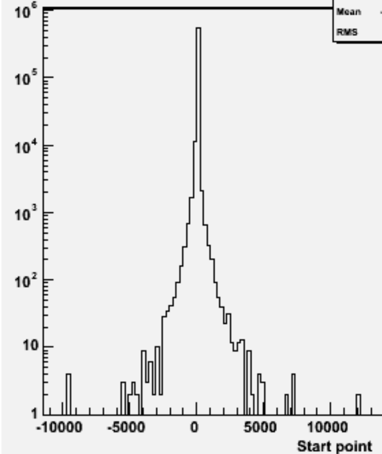
Start point Z : w104370 e1e1h_o
