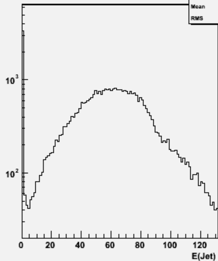
Jet energies(All jets)w104370 e1e1h_o
