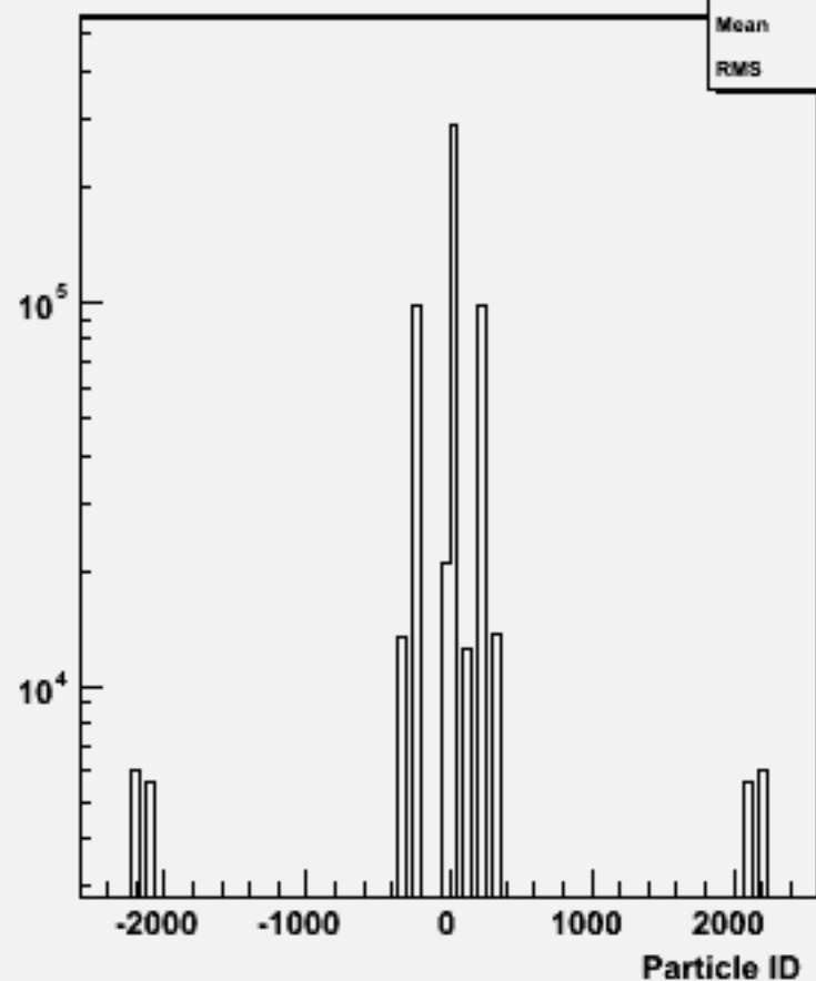
Particle ID : w104370 e1e1h_o
