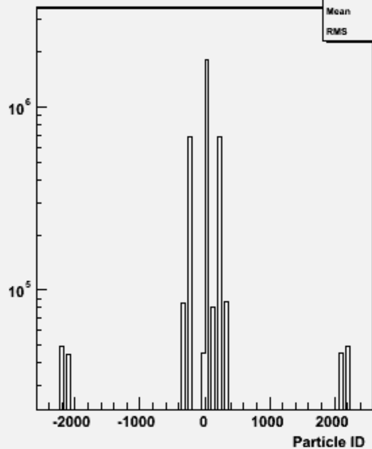
Particle ID : w104364 uuh_o
