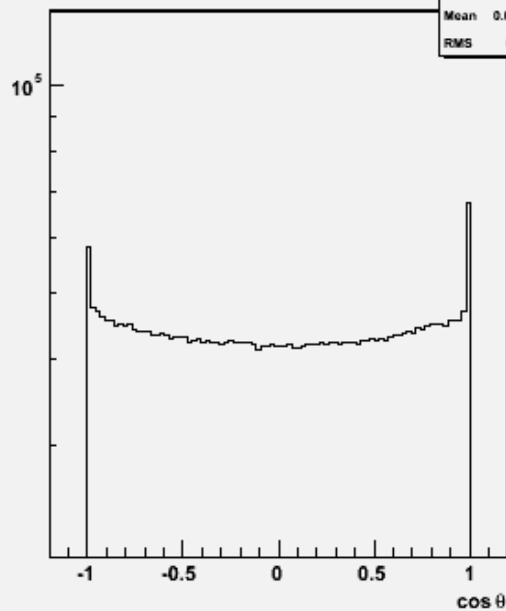
Particle cosθ : w104364 uuh_o
