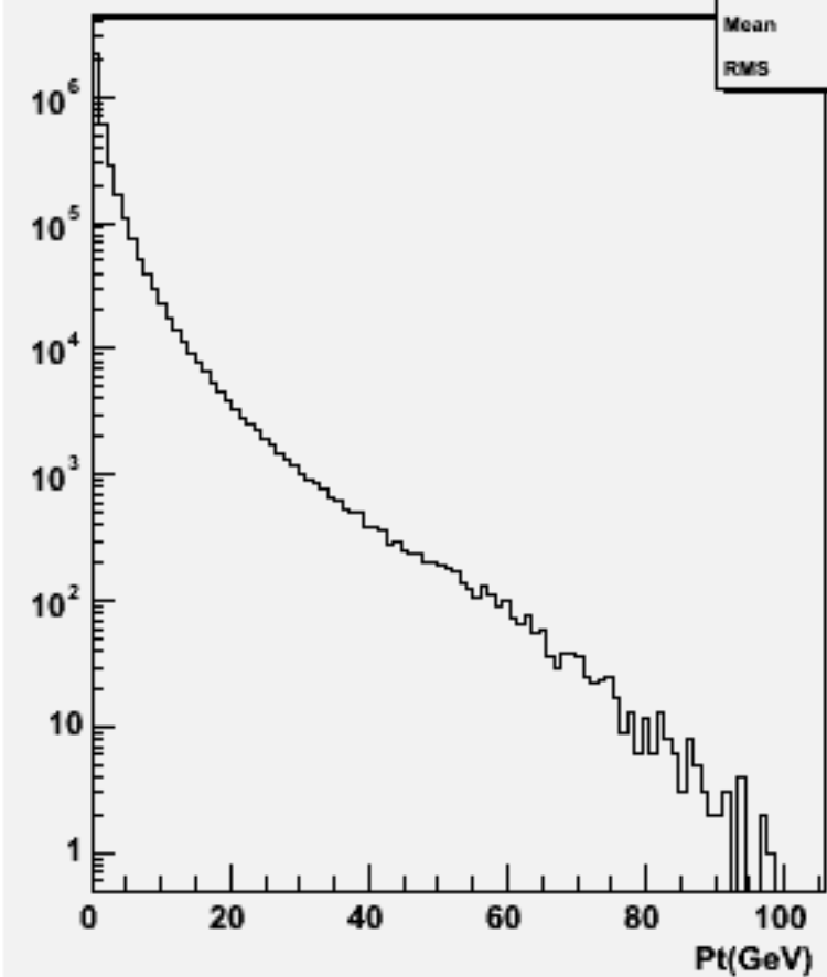
Particle Pt : w104364 uuh_o
