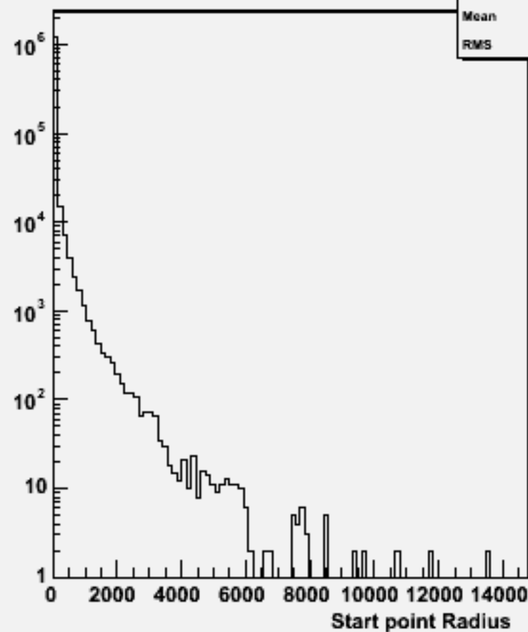
Start point R : w104360 n3n3h_o
