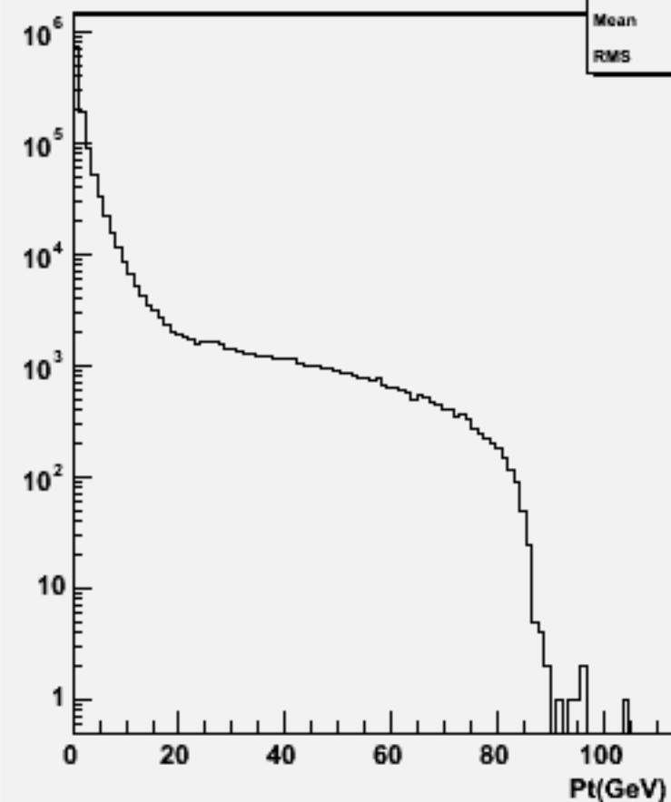
Particle Pt : w104360 n3n3h_o
