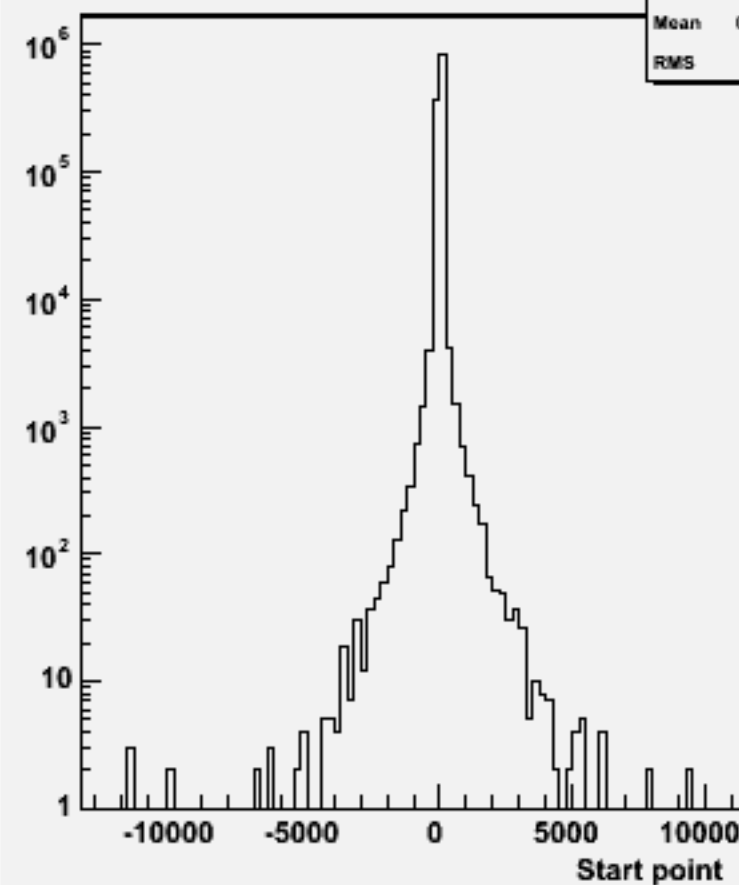
Start point Z : w104360 n3n3h_o
