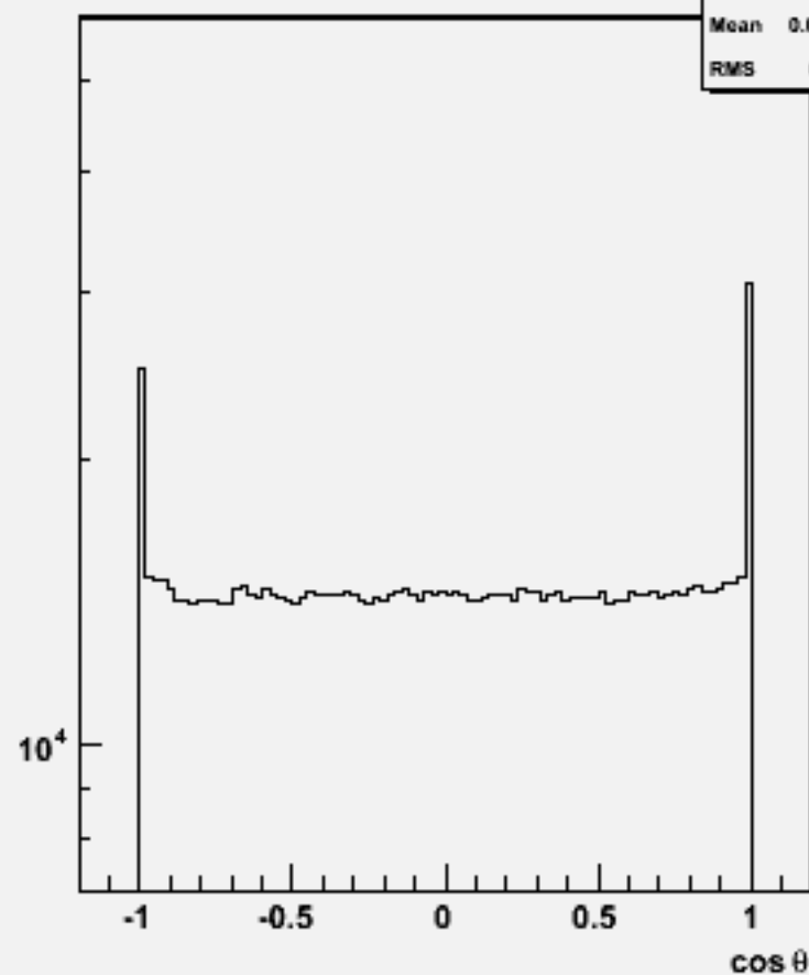
Particle cos \theta : w104360 n3n3h_o
