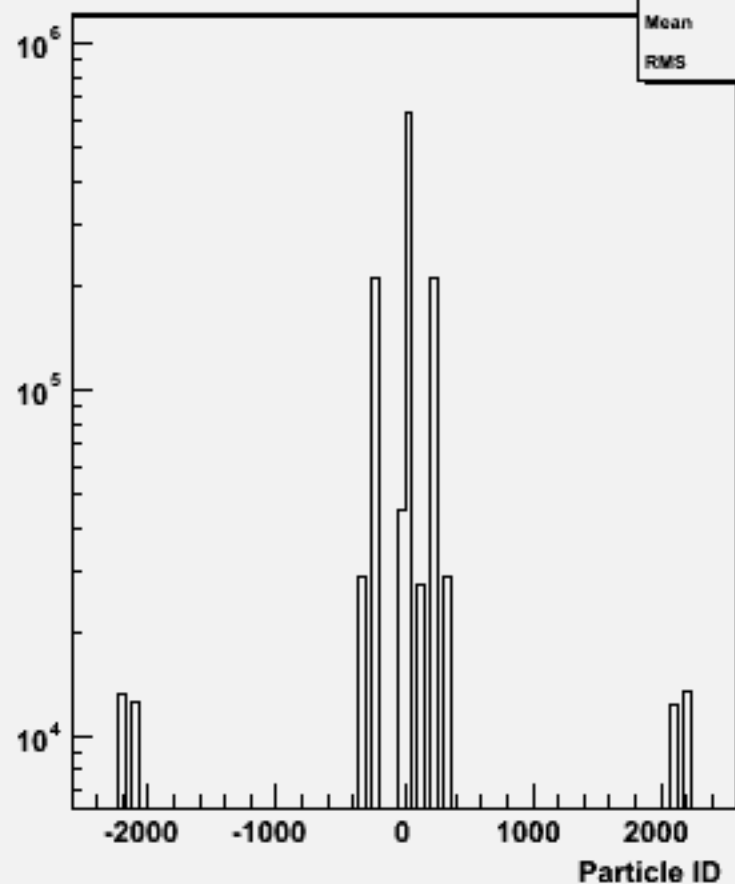
Particle ID : w104360 n3n3h_o
