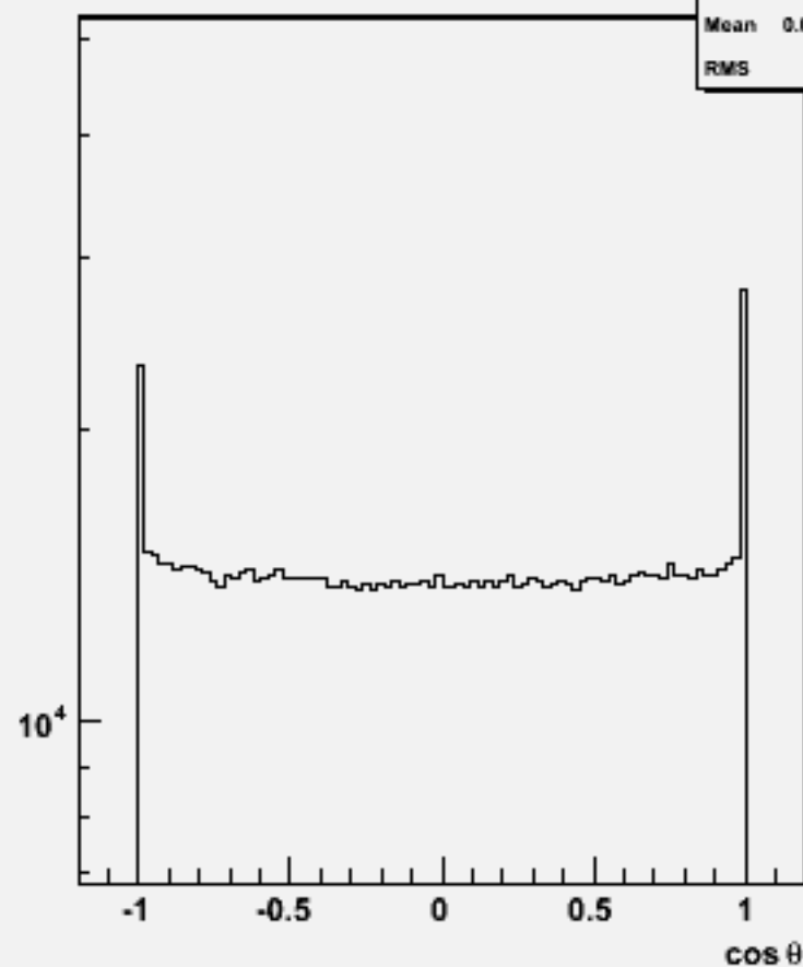
Particle cosθ : w104329 e3e3h_o
