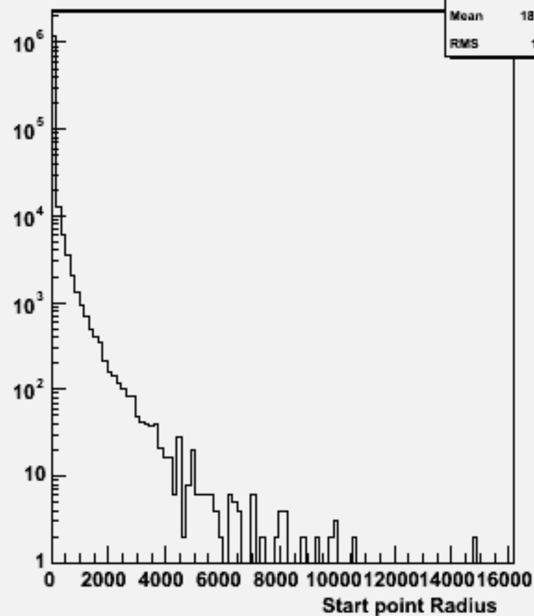
Start point R : w104329 e3e3h_o
