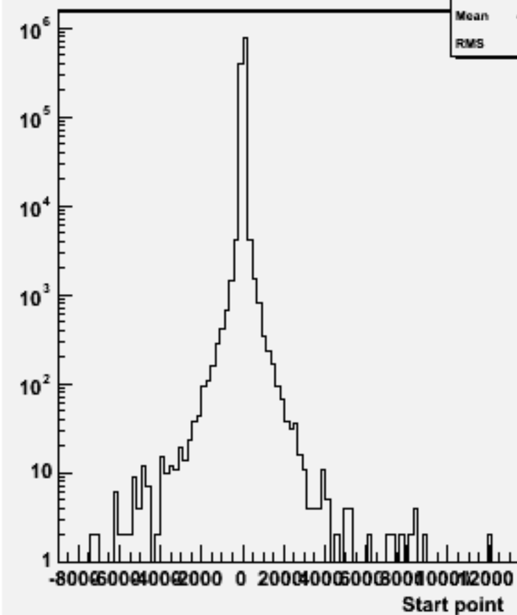
Start point Z : w104329 e3e3h_o
