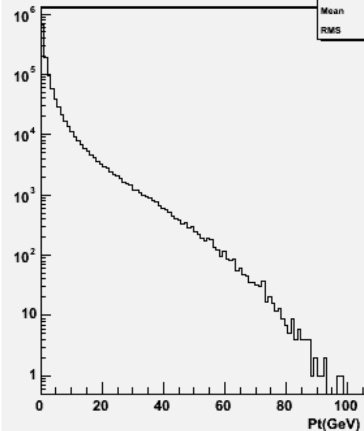
Particle Pt : w104329 e3e3h_o
