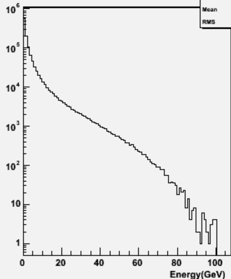
Particle Energy : w104329 e3e3h_o
