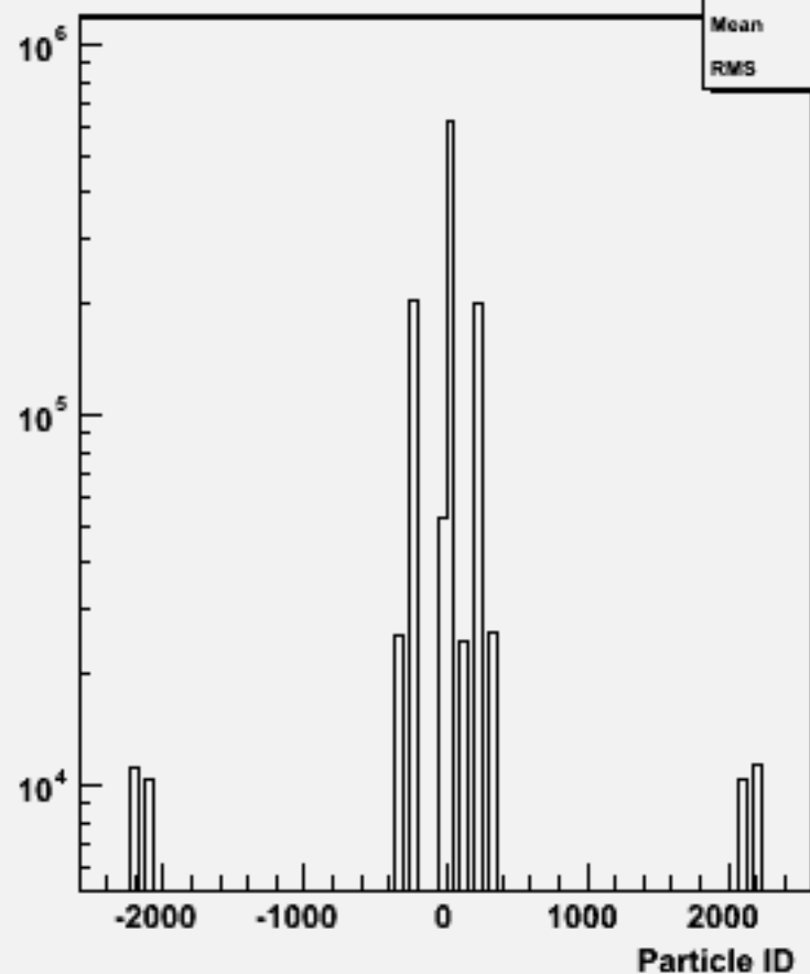
Particle ID : w104329 e3e3h_o
