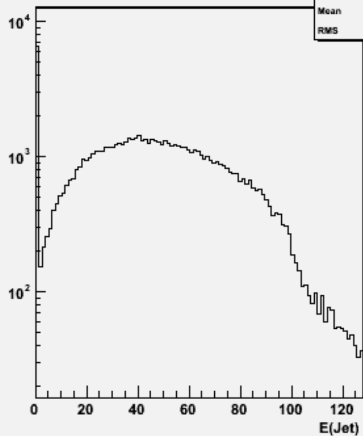
Jet energies(All jets)w104329 e3e3h_o
