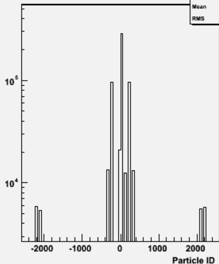
Particle ID : w104323 e1e1h_o
