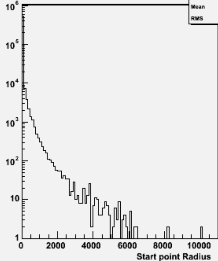
Start point R : w104323 e1e1h_o
