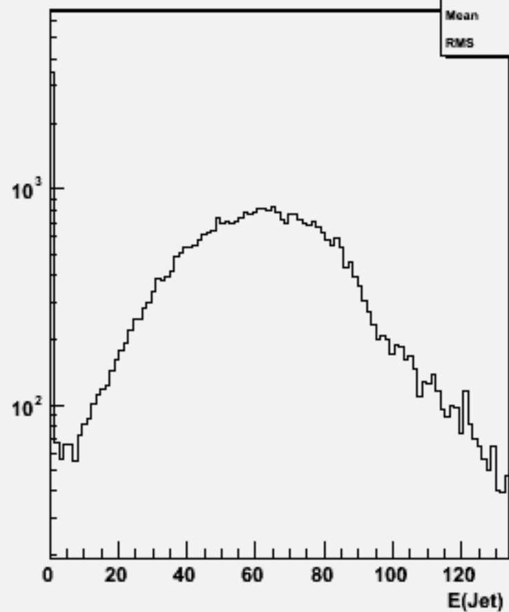
Jet energies(All jets)w104323 e1e1h_o
