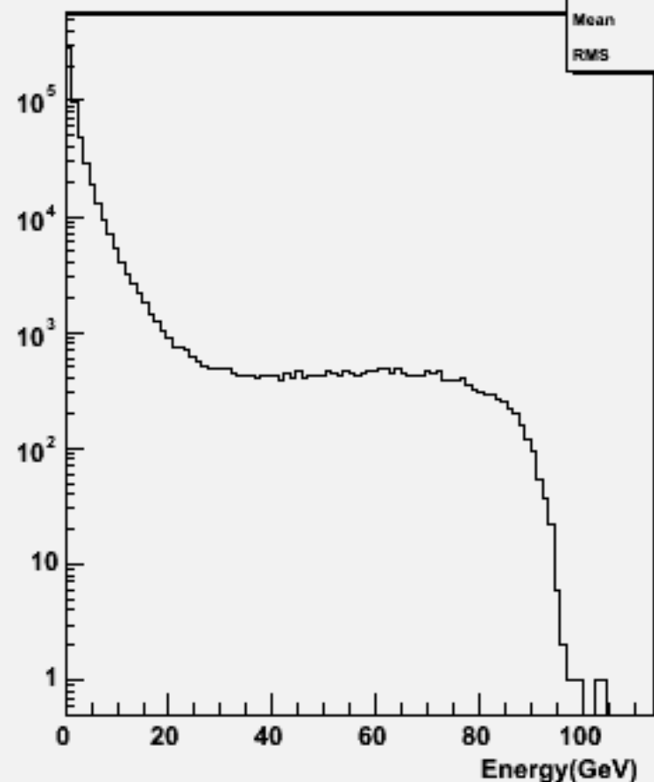
Particle Energy : w104323 e1e1h_o
