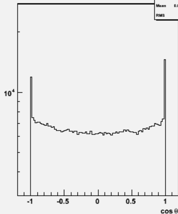
Particle cosθ : w104323 e1e1h_o
