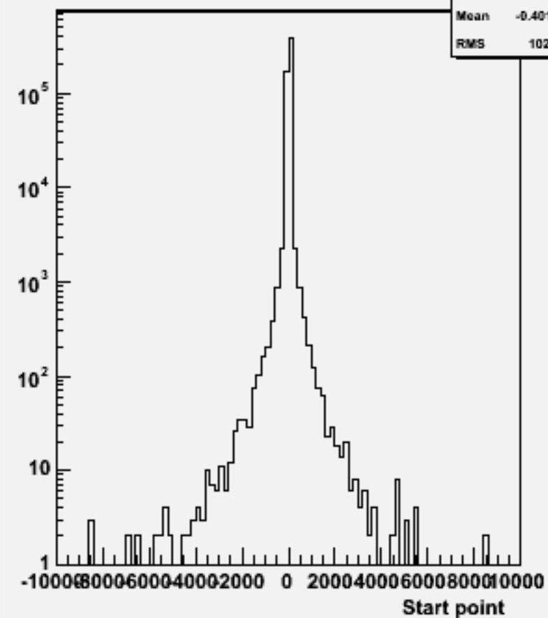
Start point Z : w104323 e1e1h_o
