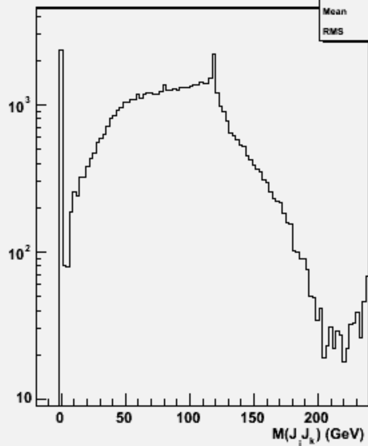
2jets mass(All comb)w104323 e1e1h_o
