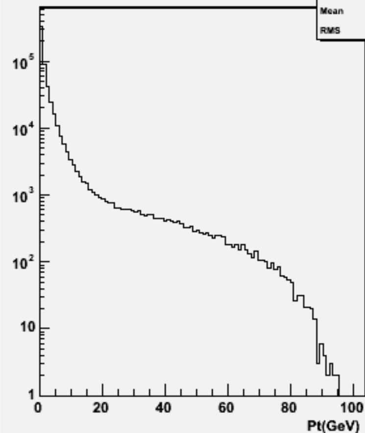
Particle Pt : w104323 e1e1h_o
