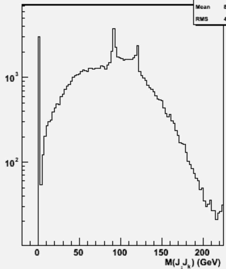
2jets mass(All comb)w104322 e1e1h_o
