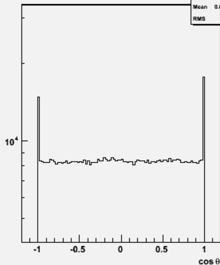
Particle cos \theta : w104322 e1e1h_o
