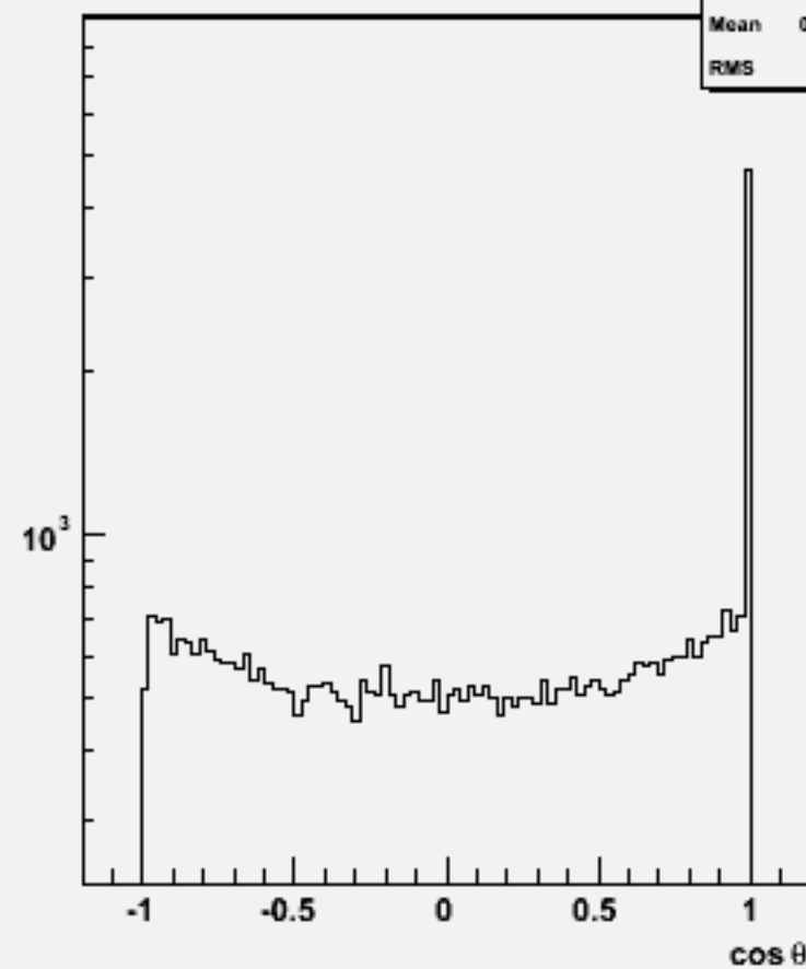
Jet cos \theta (All jets)w104322 e1e1h_o
