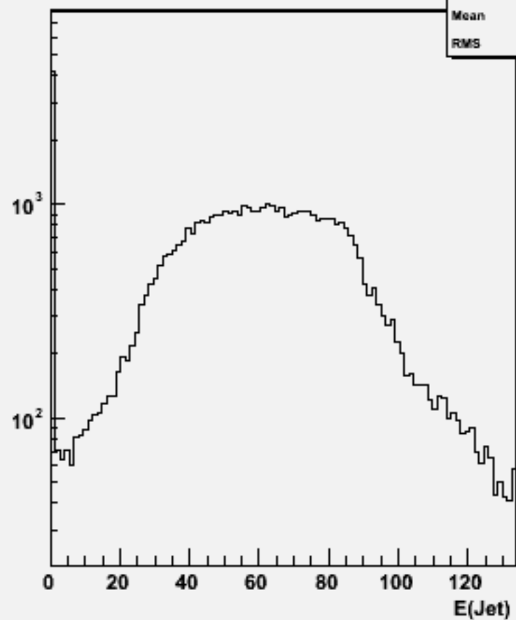
Jet energies(All jets)w104322 e1e1h_o
