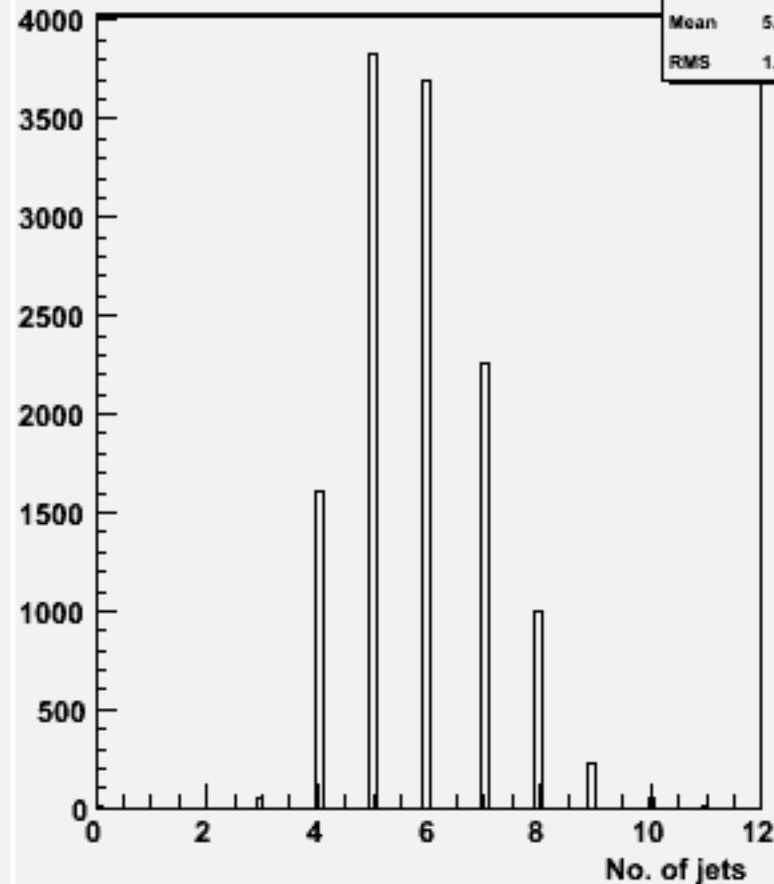
No. jets (ycut=0.001) : w104322 e1e1h_o
