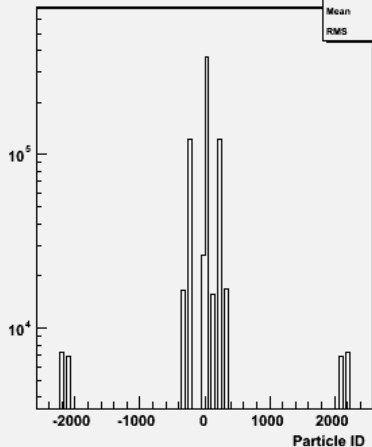
Particle ID : w104322 e1e1h_o
