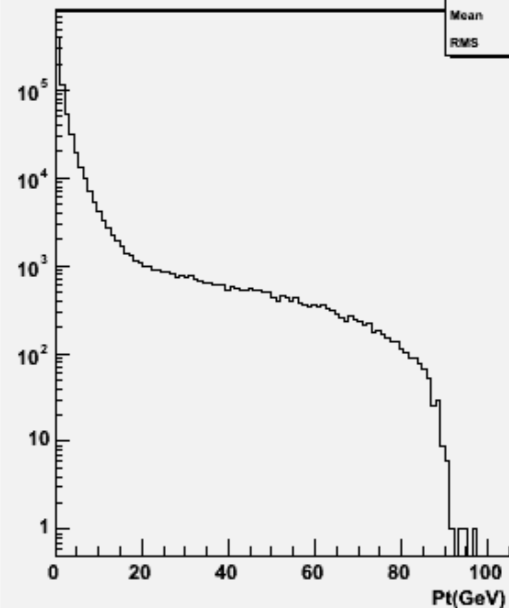
Particle Pt : w104322 e1e1h_o
