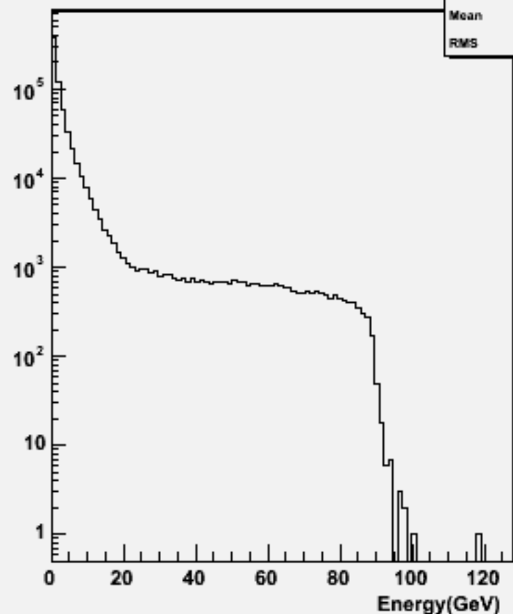
Particle Energy : w104322 e1e1h_o
