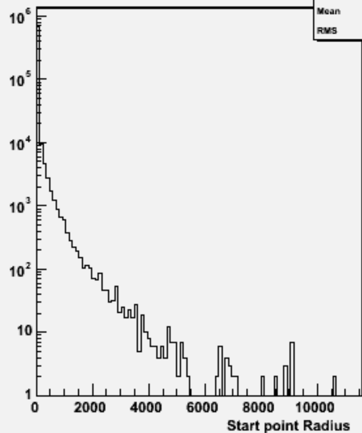
Start point R : w104322 e1e1h_o
