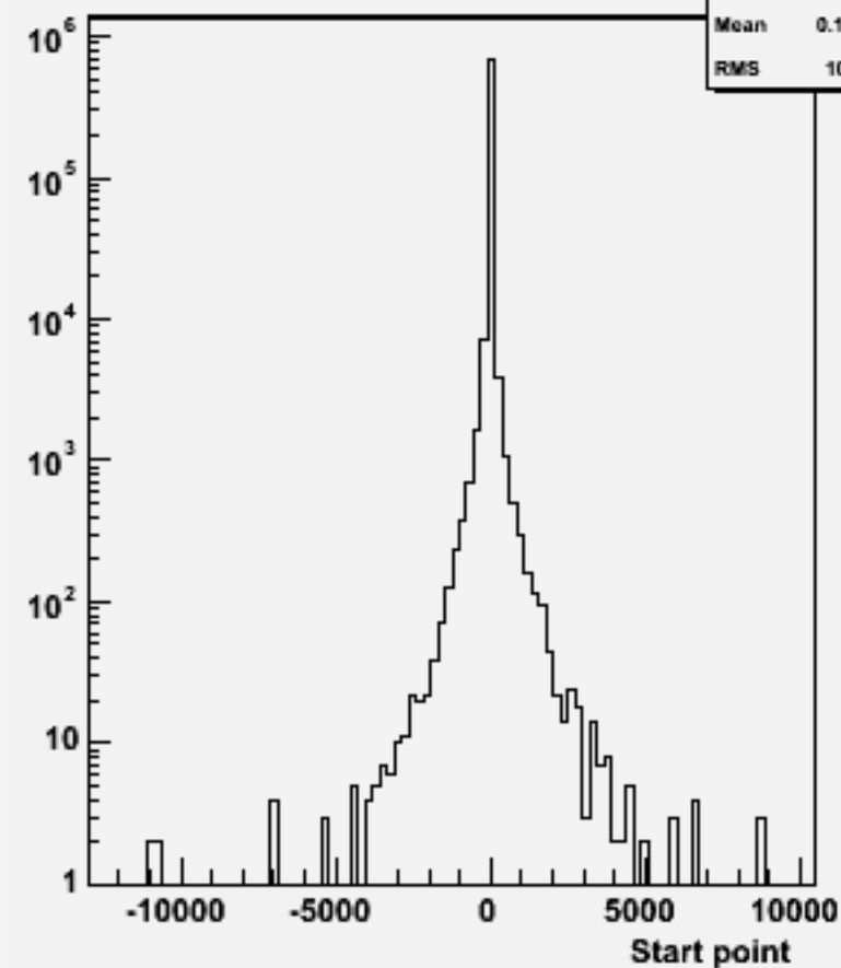
Start point Z : w104322 e1e1h_o
