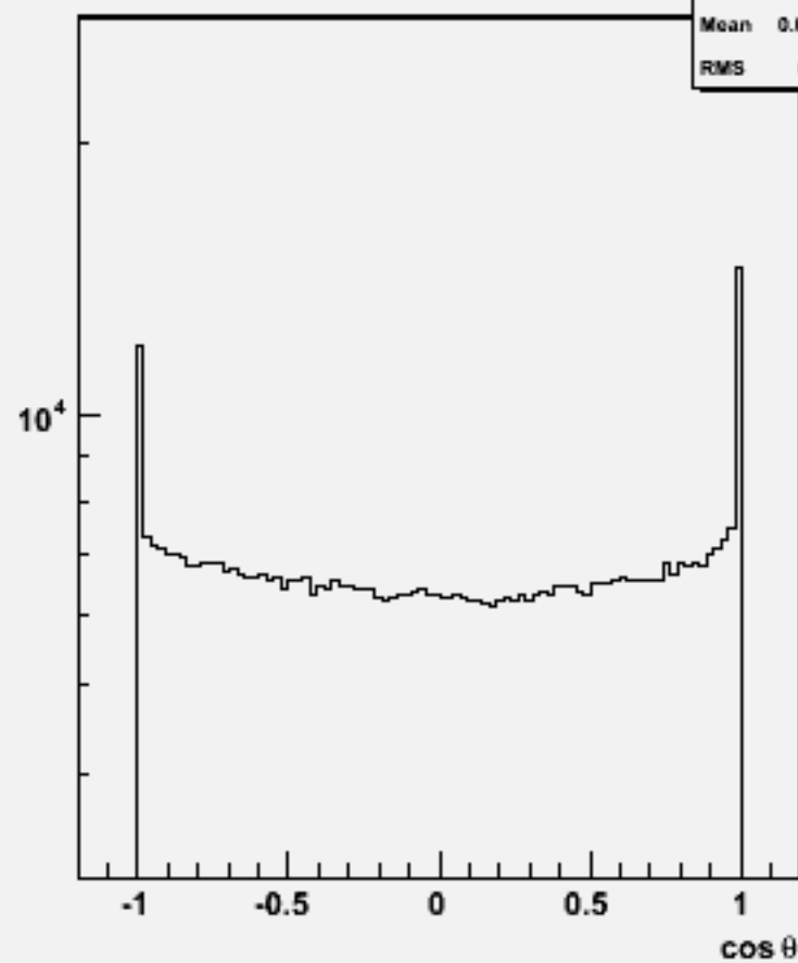
Particle cosθ : w104320 e1e1h_o
