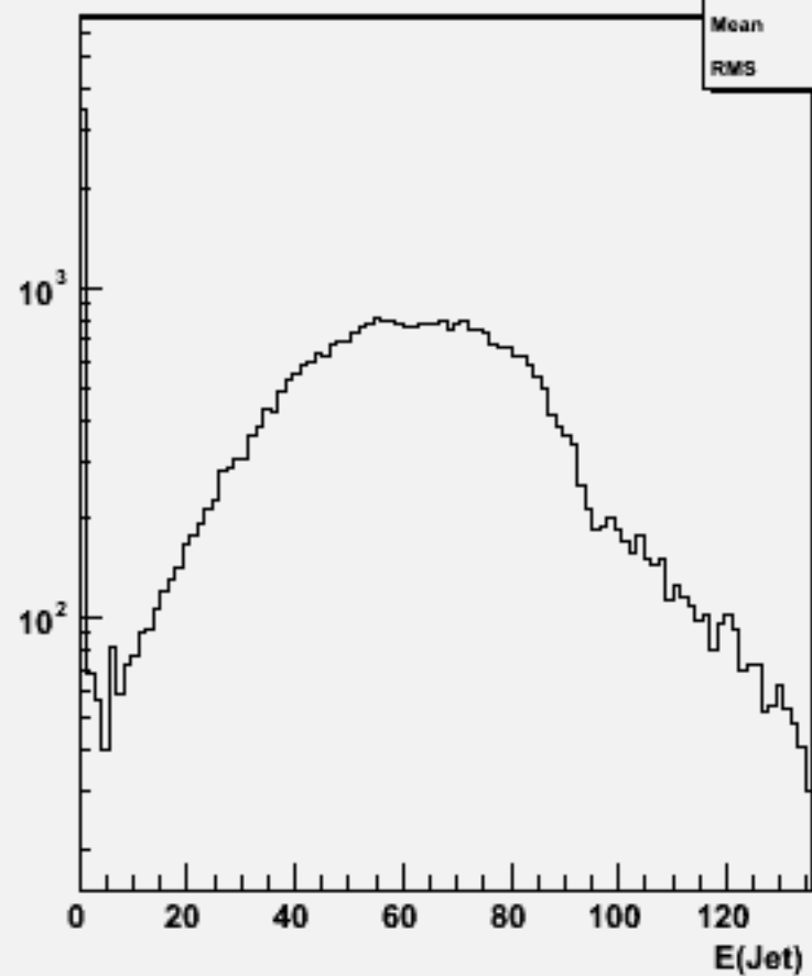
Jet energies(All jets)w104320 e1e1h_o
