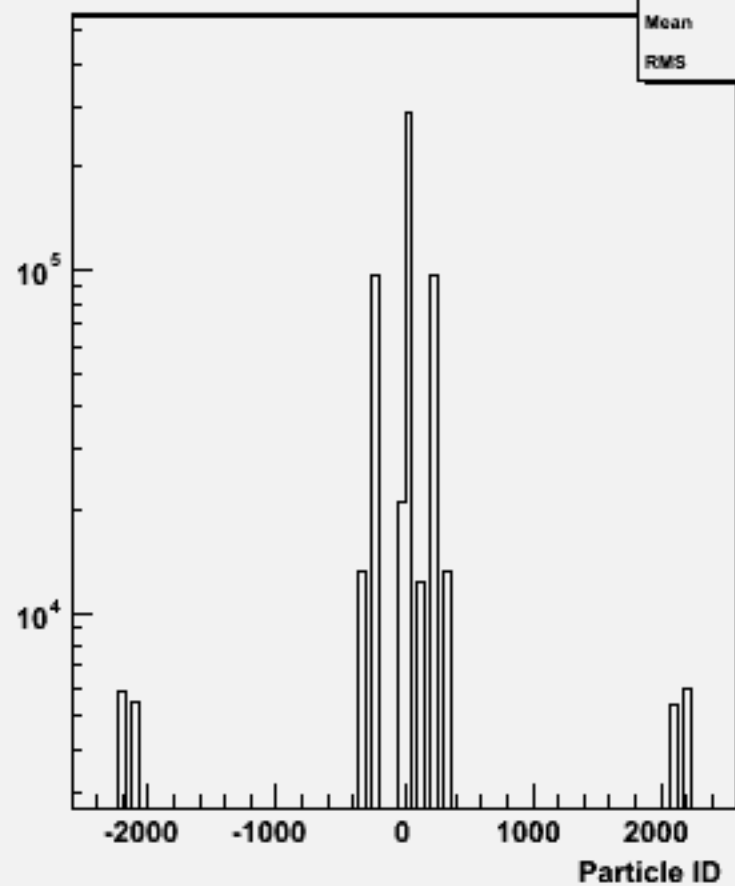
Particle ID : w104320 e1e1h_o
