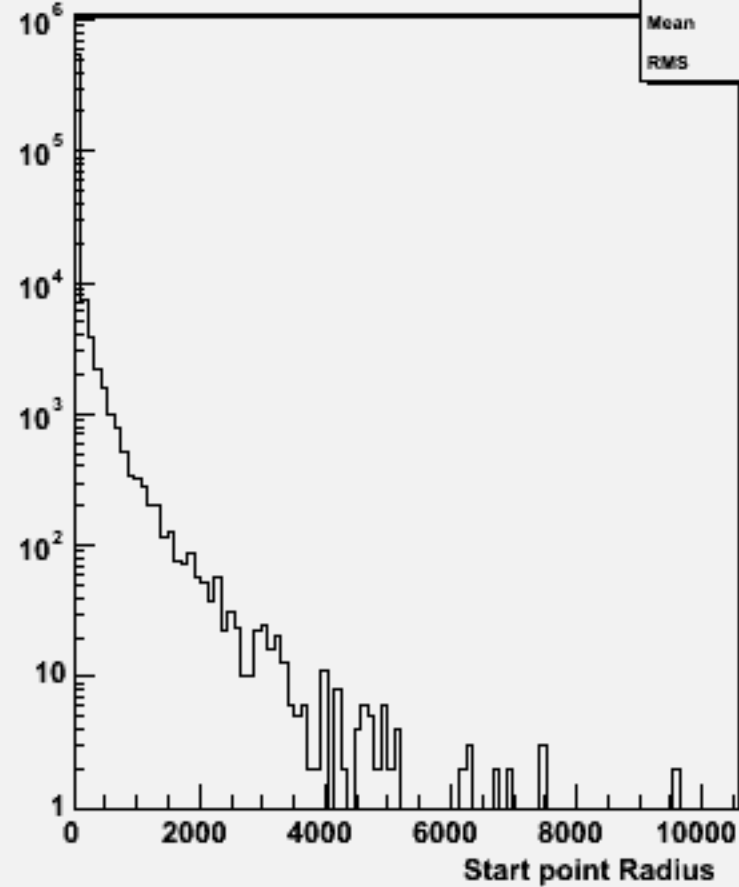
Start point R : w104320 e1e1h_o
