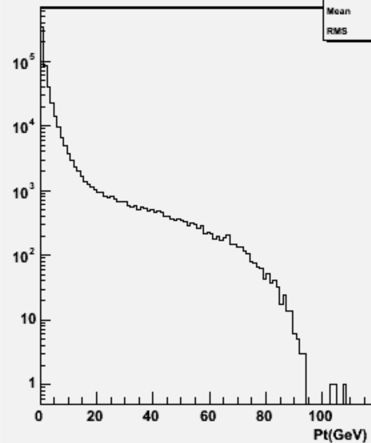
Particle Pt : w104320 e1e1h_o
