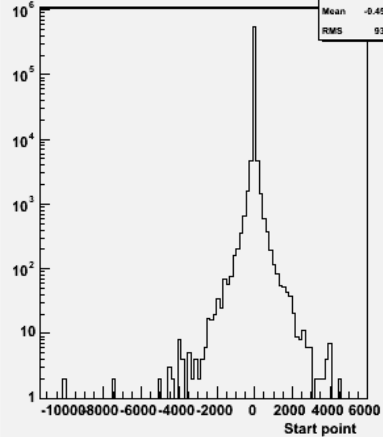
Start point Z : w104320 e1e1h_o
