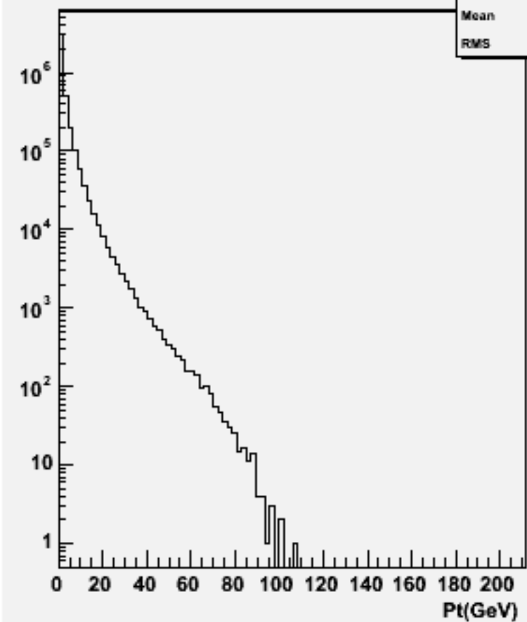
Particle Pt : w104314 uuh_o
