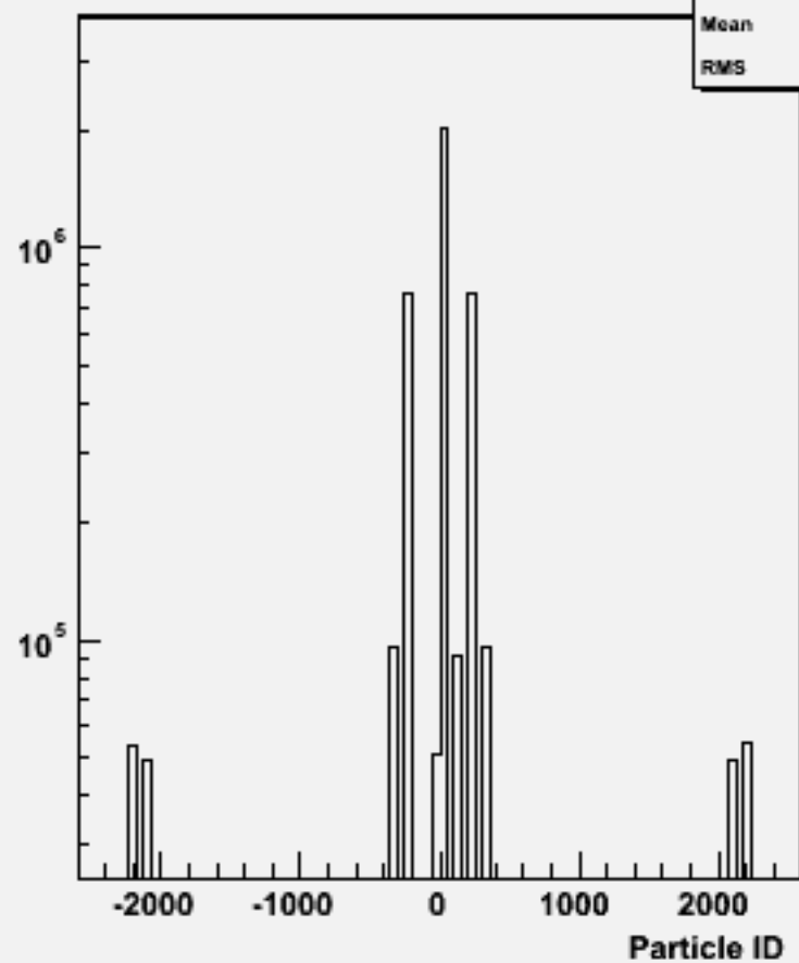
Particle ID : w104314 uuh_o
