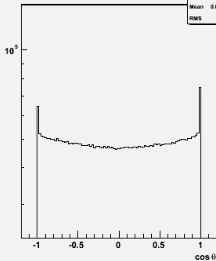
Particle cosθ : w104314 uuh_o
