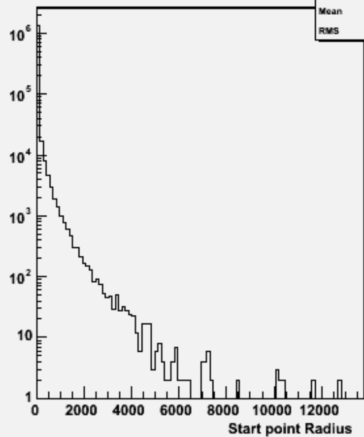
Start point R : w104310 n3n3h_o
