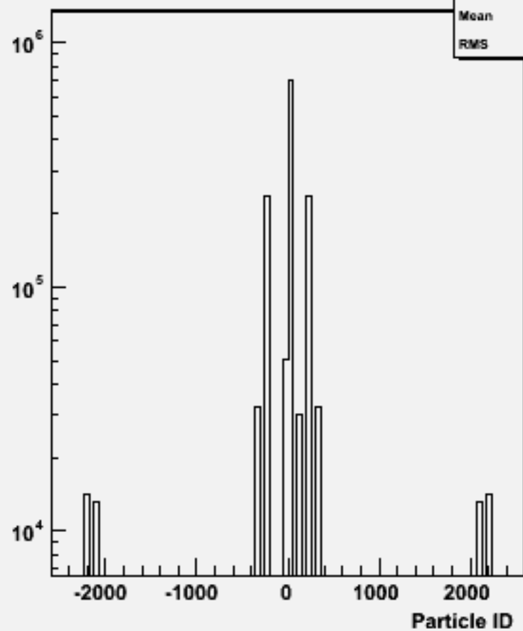
Particle ID : w104310 n3n3h_o
