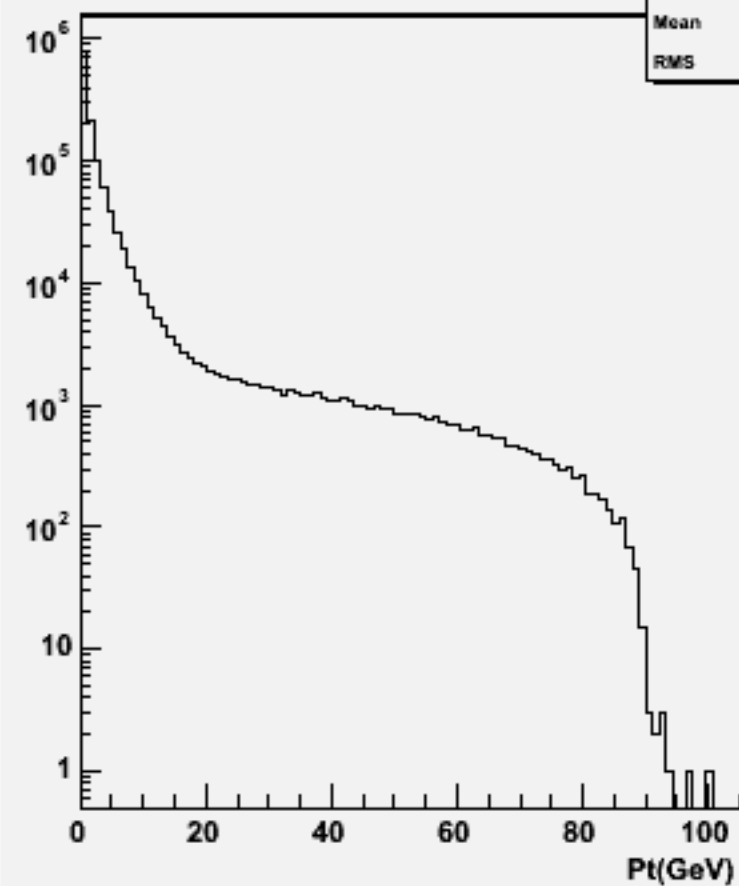
Particle Pt : w104310 n3n3h_o
