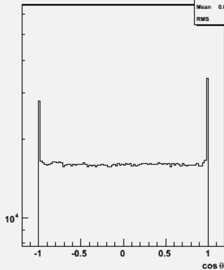
Particle \cos\theta : w104310 n3n3h_o
