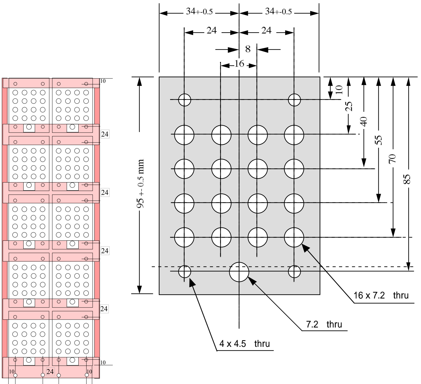
参考図 パネルフレームとの 組上げ状態図
