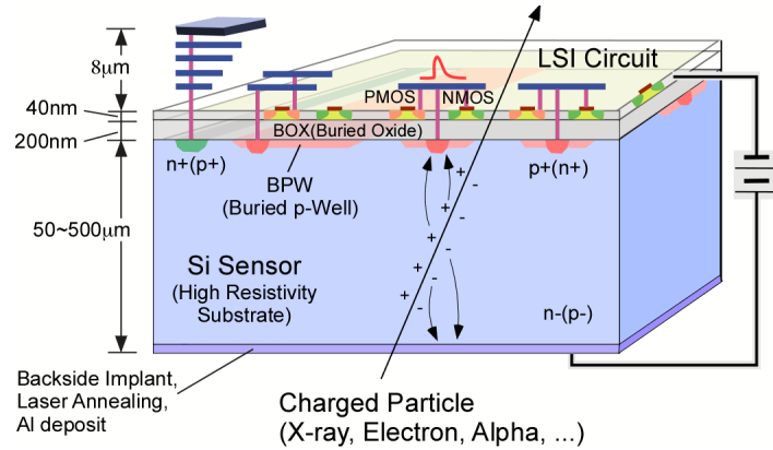
図 2. SOI 検出器の構造
